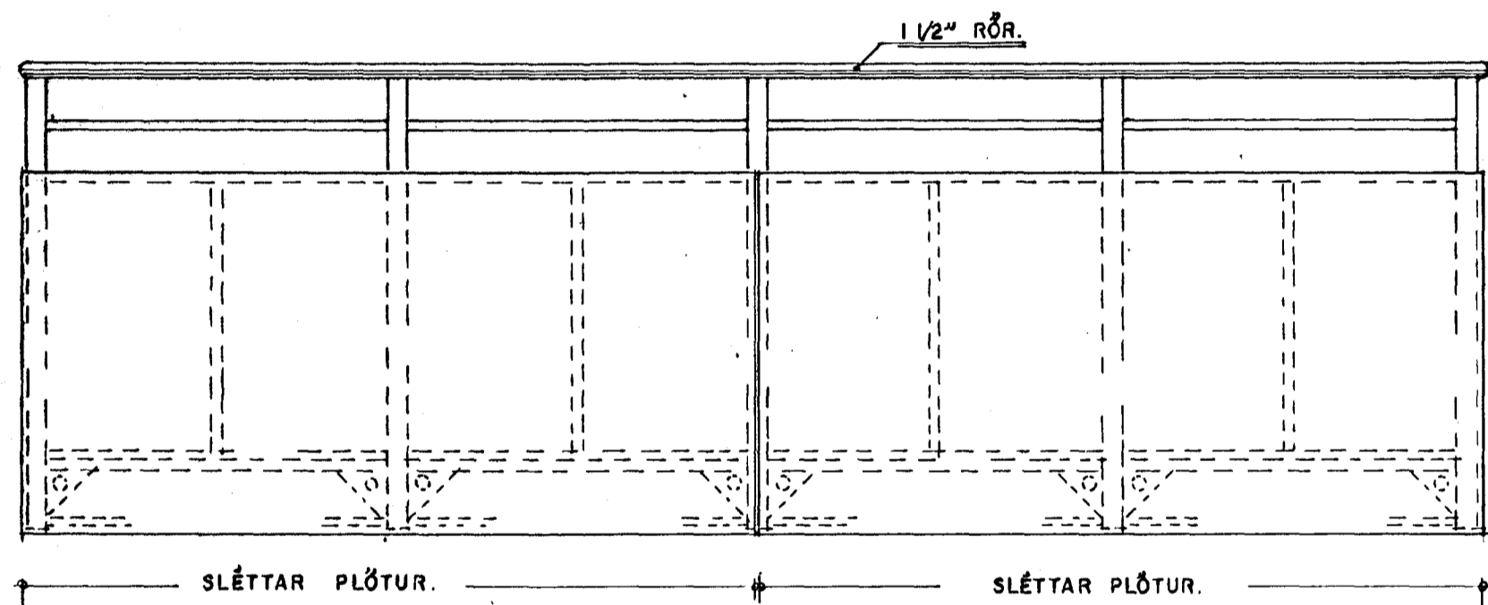
SÉÐ FRAMANÁ SVALIR Á VESTURHLIÐ. 1:20
