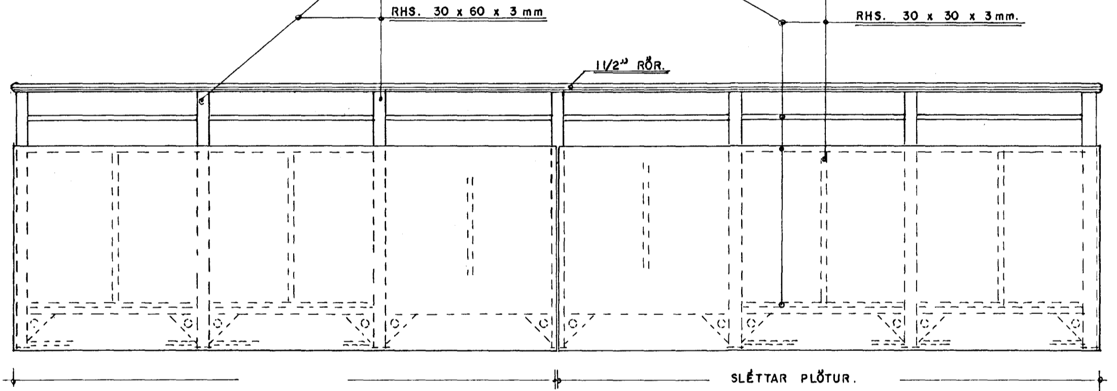
SÉÐ FRAMANÁ SVALIR Á SUÐURHLIÐ. 1:20
