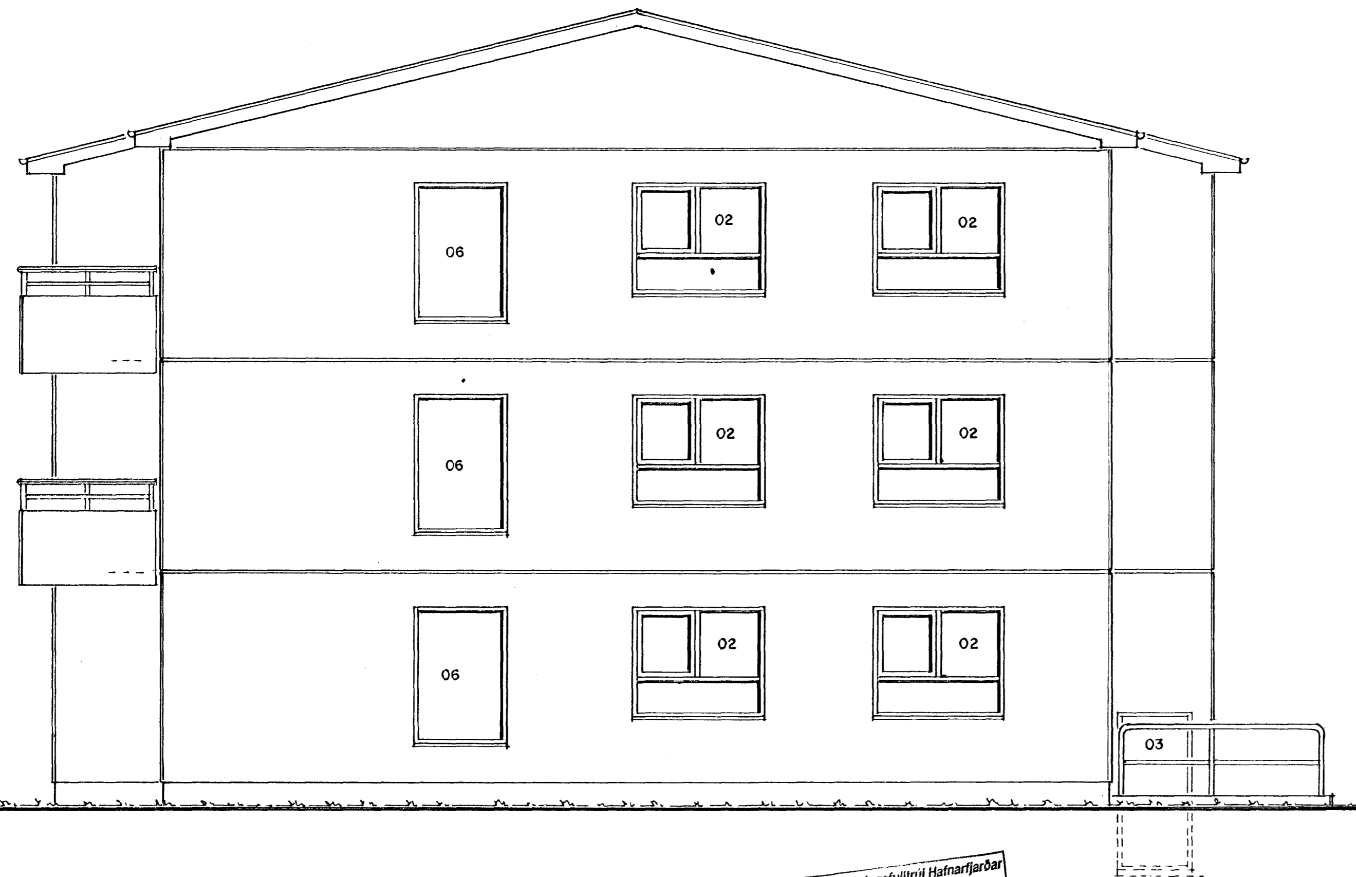
AUSTURHLIÐ. 1:50
