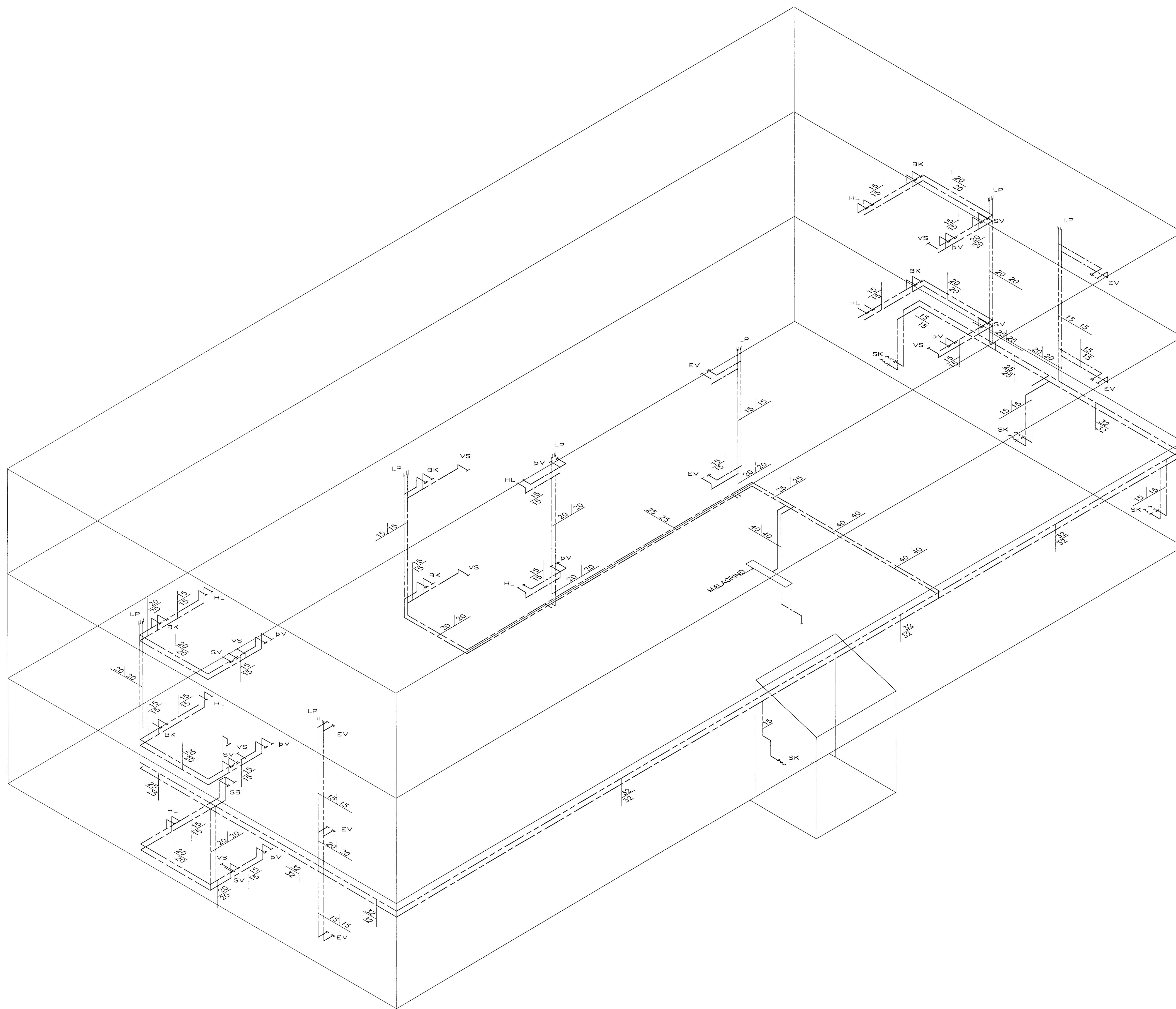
RÚMMYND VATNSLAGNA 1:50
