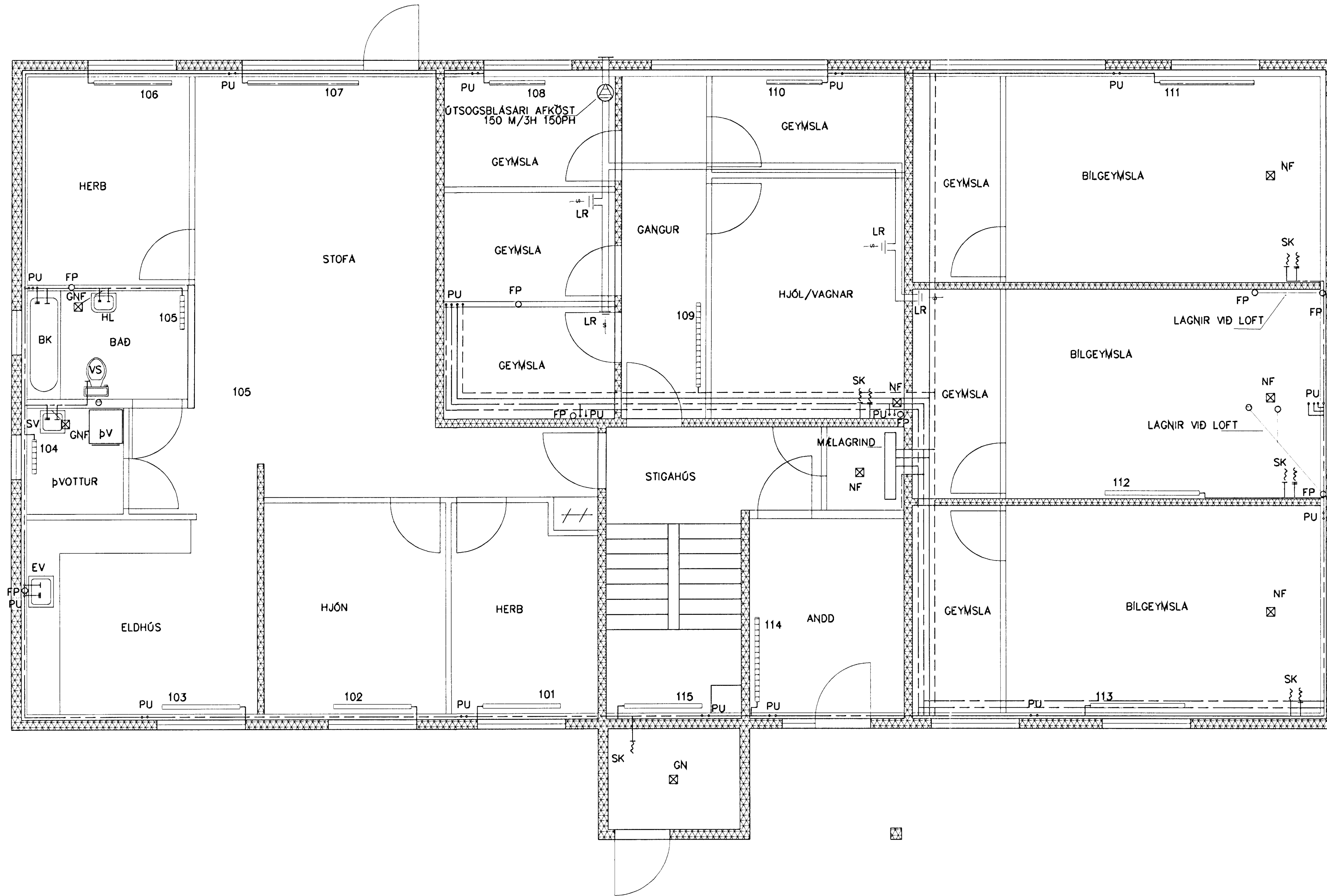
GRUNNMYND 1 HÆÐAR 1:50
