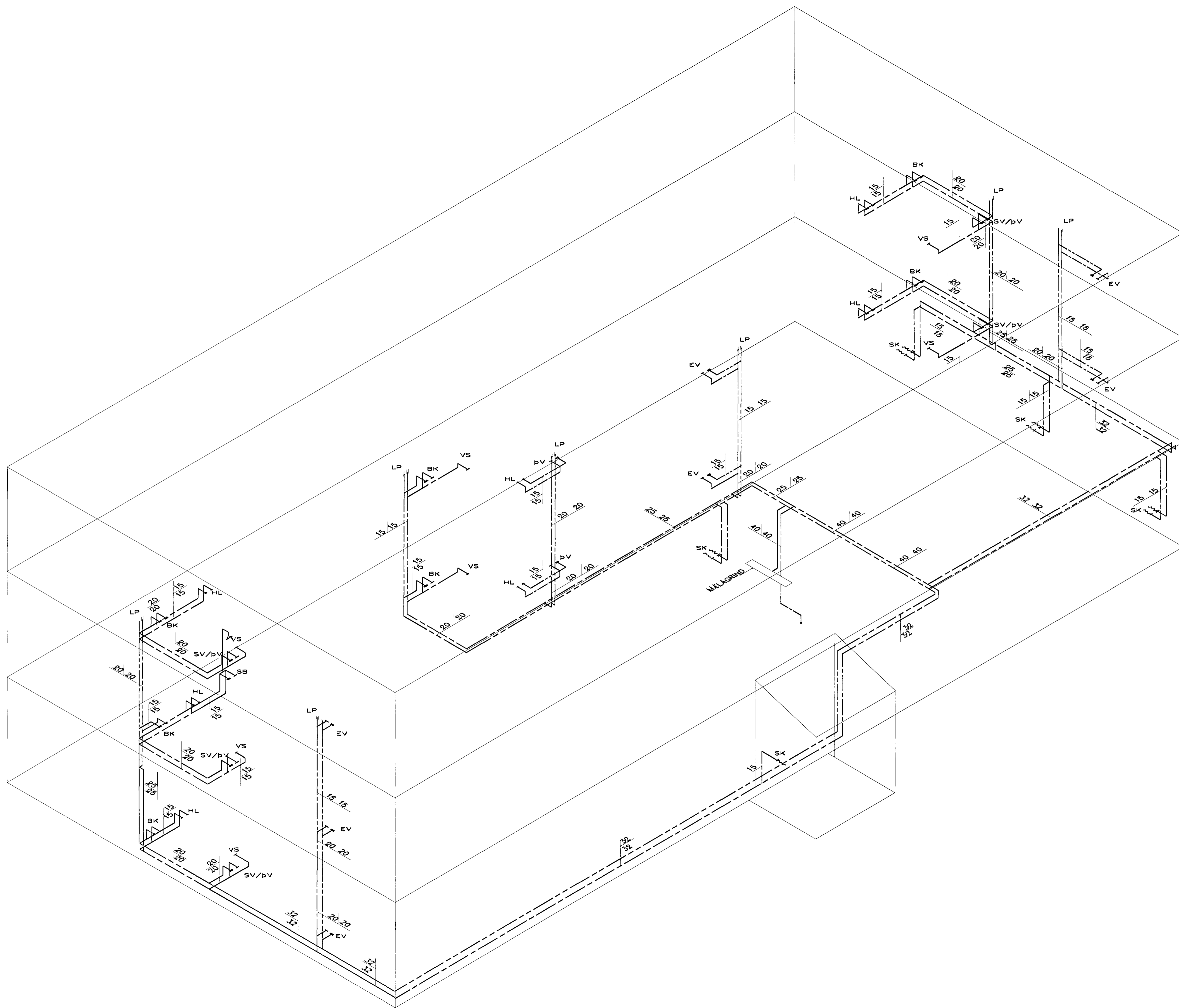
RÚMMYND VATNSLAGNA 1:50
