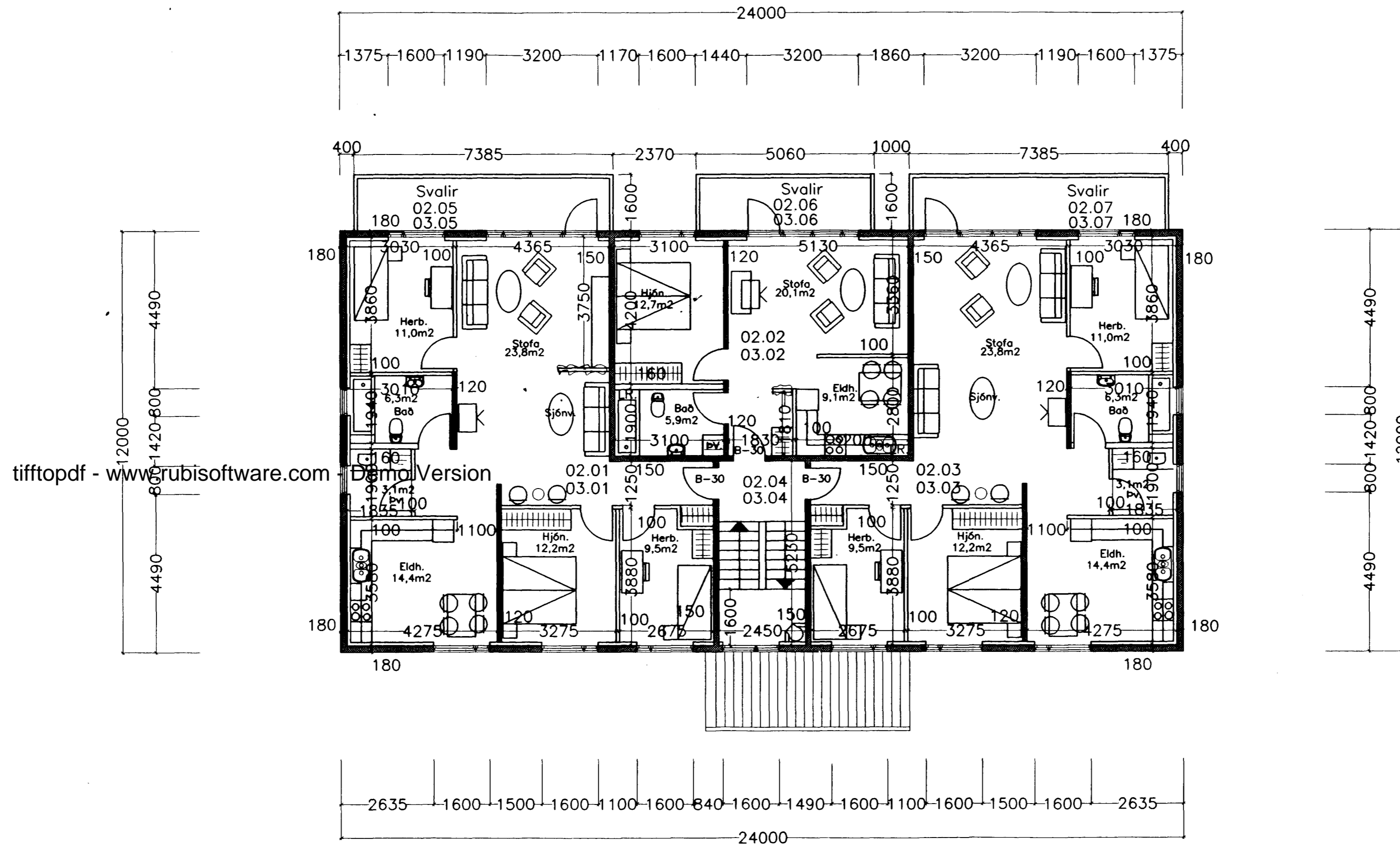
Grunnmynd 2-3 Hæðar
