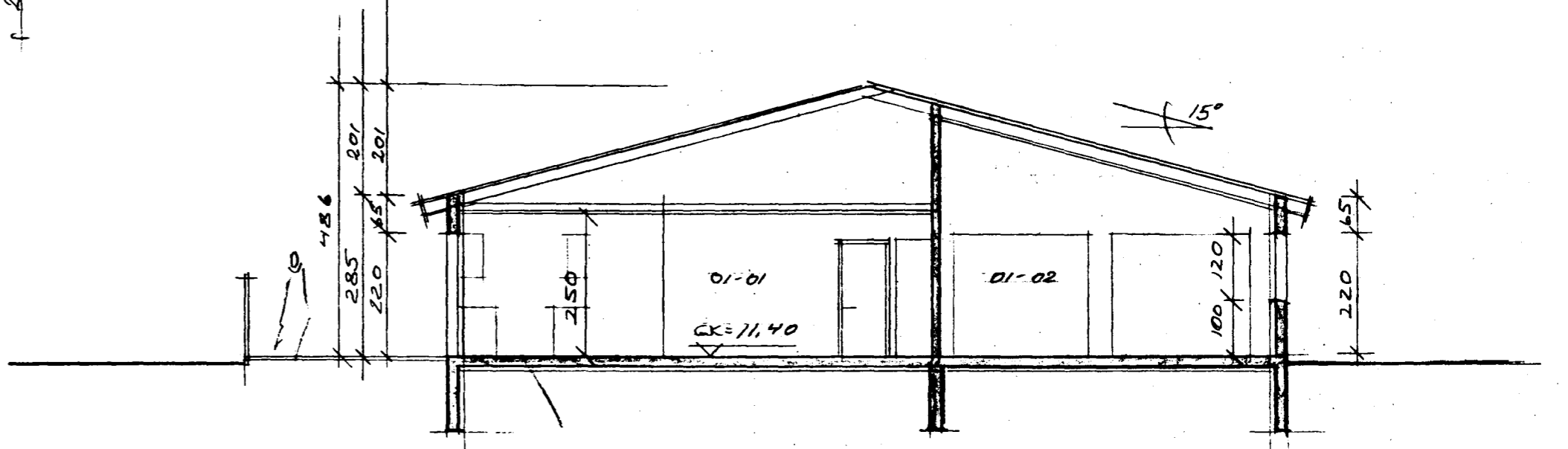
SNÍÐ A-A MKU. 1:100
