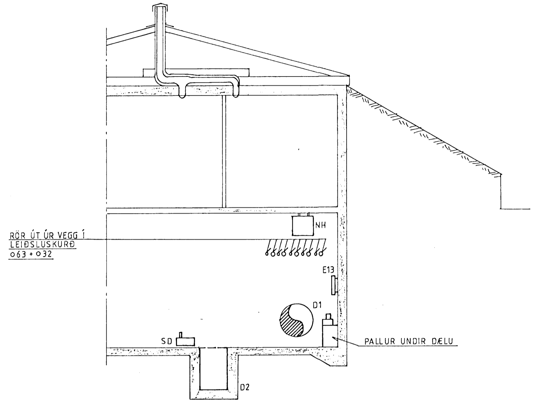
SNIÐ A-A, 1:50
