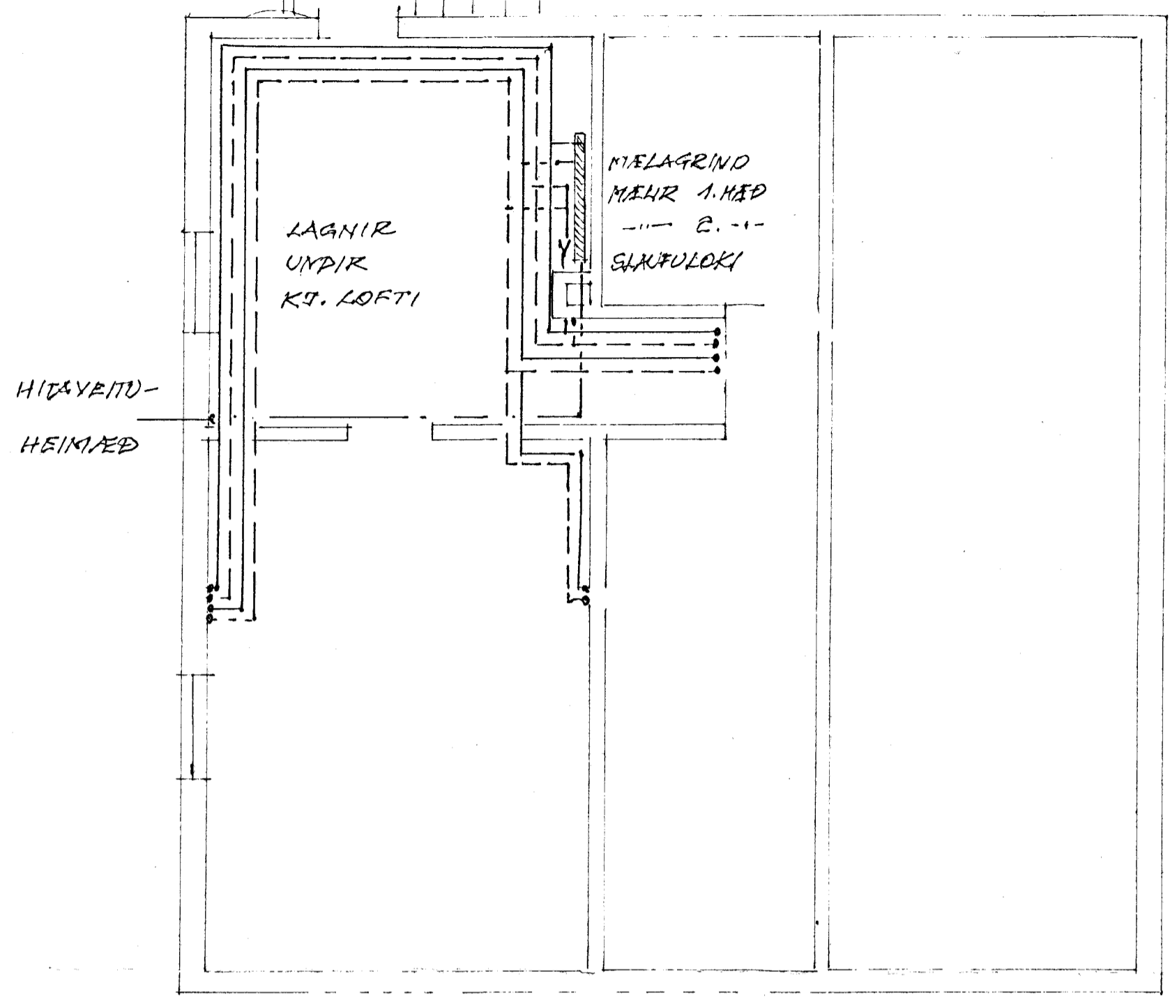
2.HÆÐ 1:50
