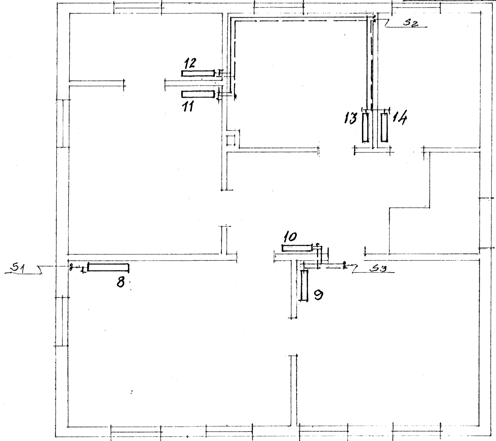
2.HÆÐ 1:50
