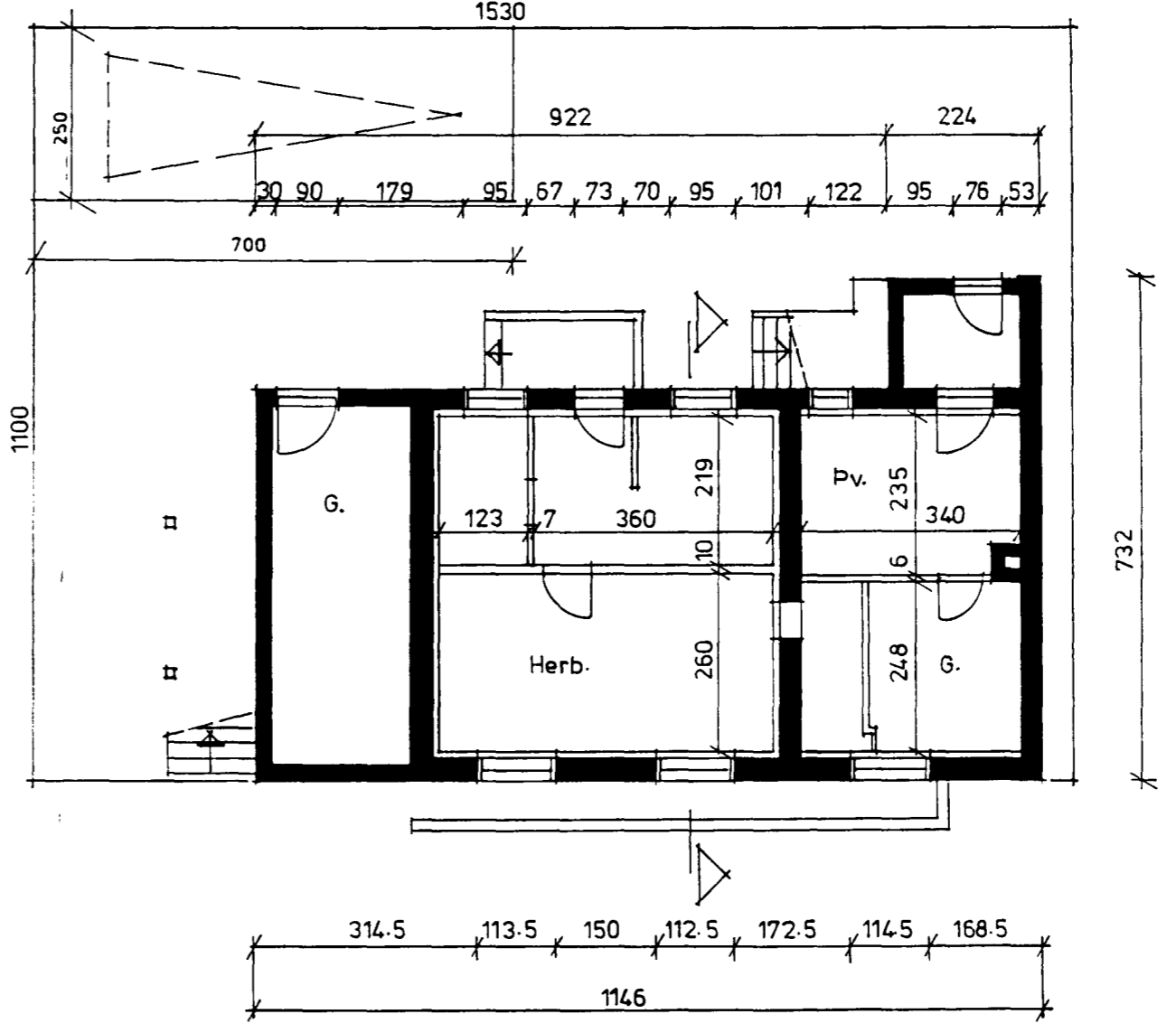
GRUNNMYND KJALLARA 1:100
