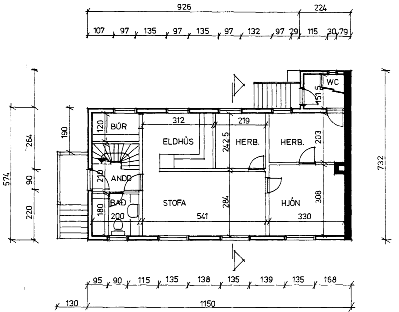
GRUNNMYND HÆÐAR 1:100
