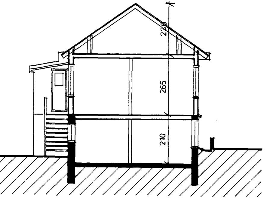
SNEIÐING
