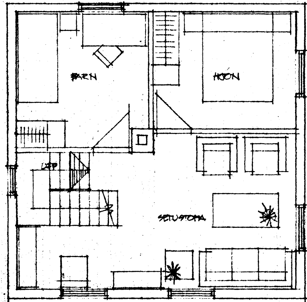
GRUNNMYND MIÐHÉÐAR 1:50
