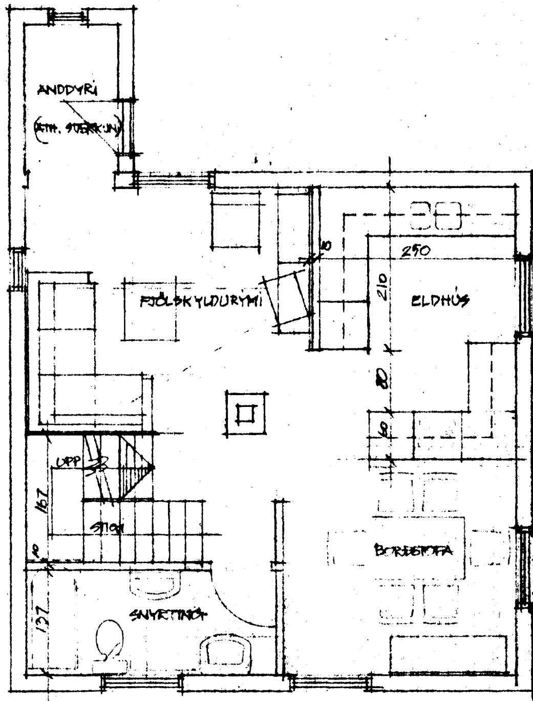
GRUNNMYND JARÐHÉÐAR 1:50
