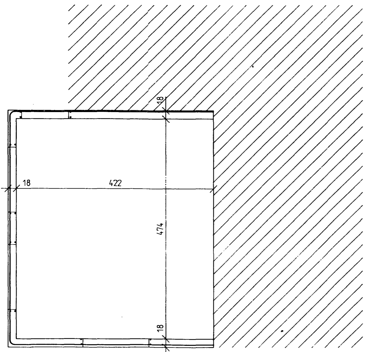
GRUNNMYND ÚTVEGGJA MKV. 1:50
