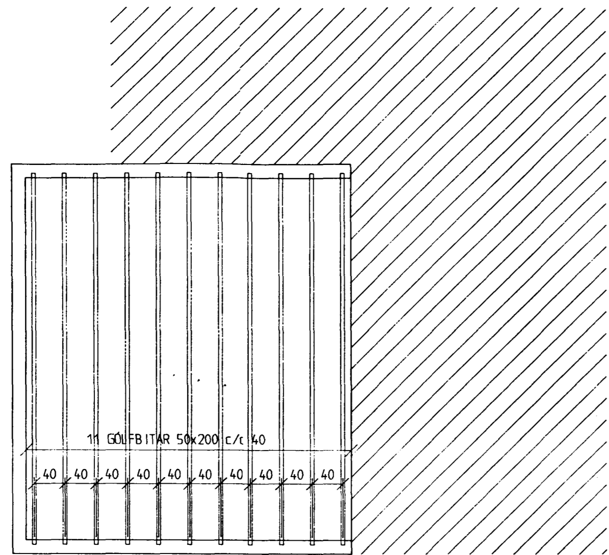
GRUNNMYND GÖLFBITA MKV. 1:50
