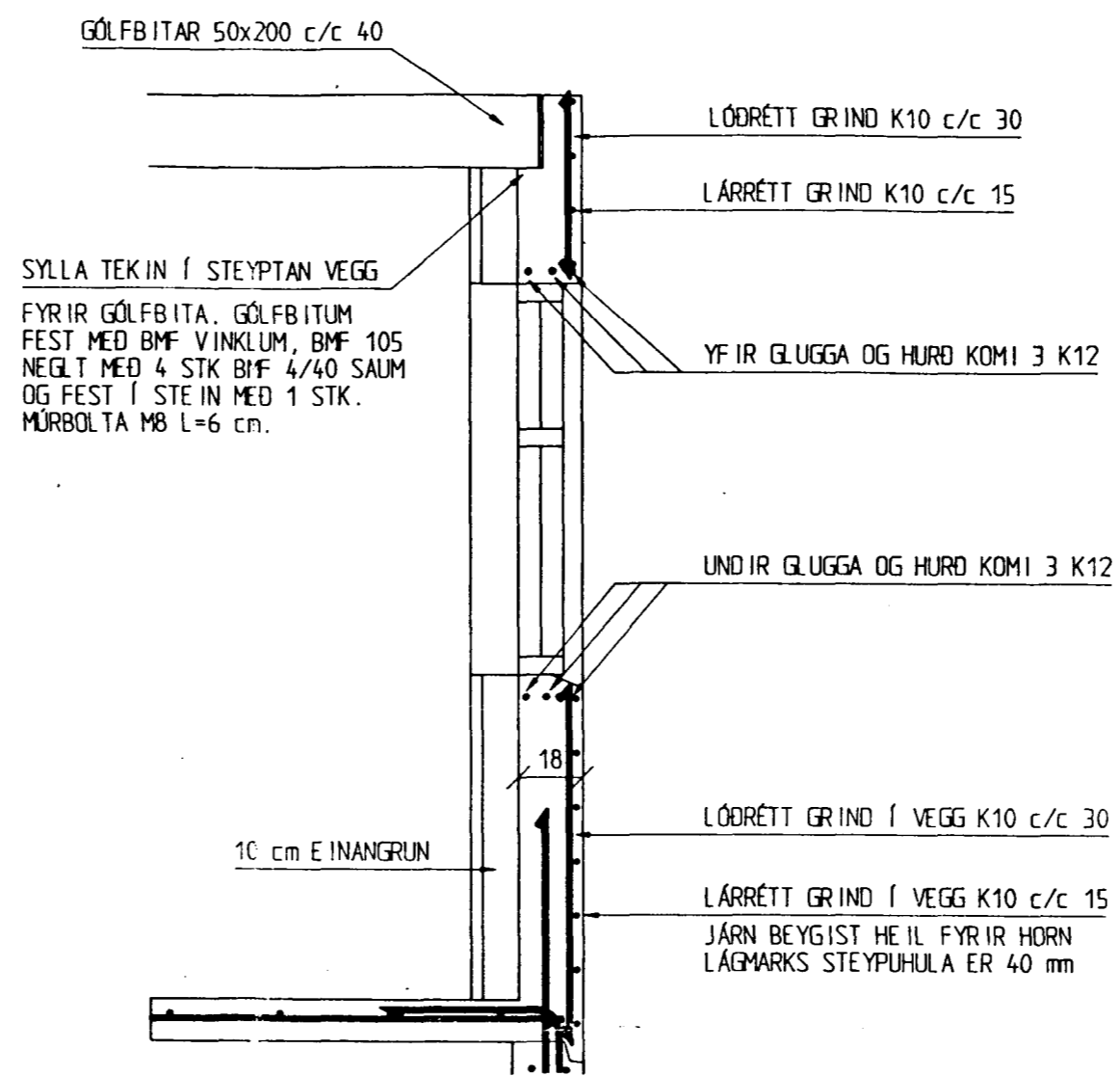
SNID Í ÚTVEGG MKV. 1:20
