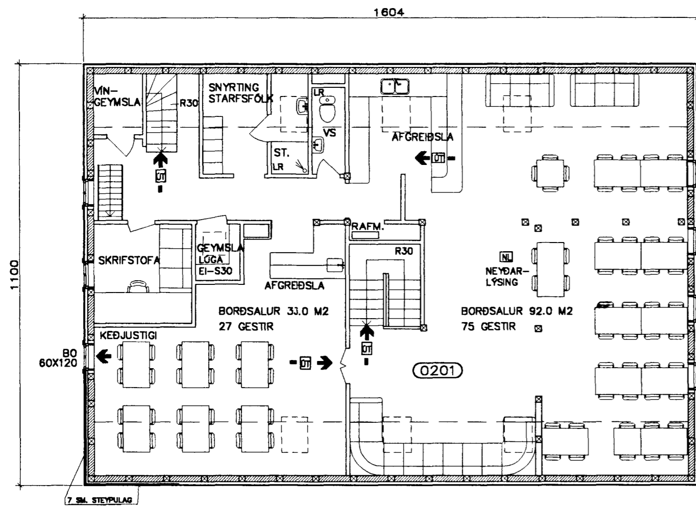
GRUNNMYND 2. HÆÐ
