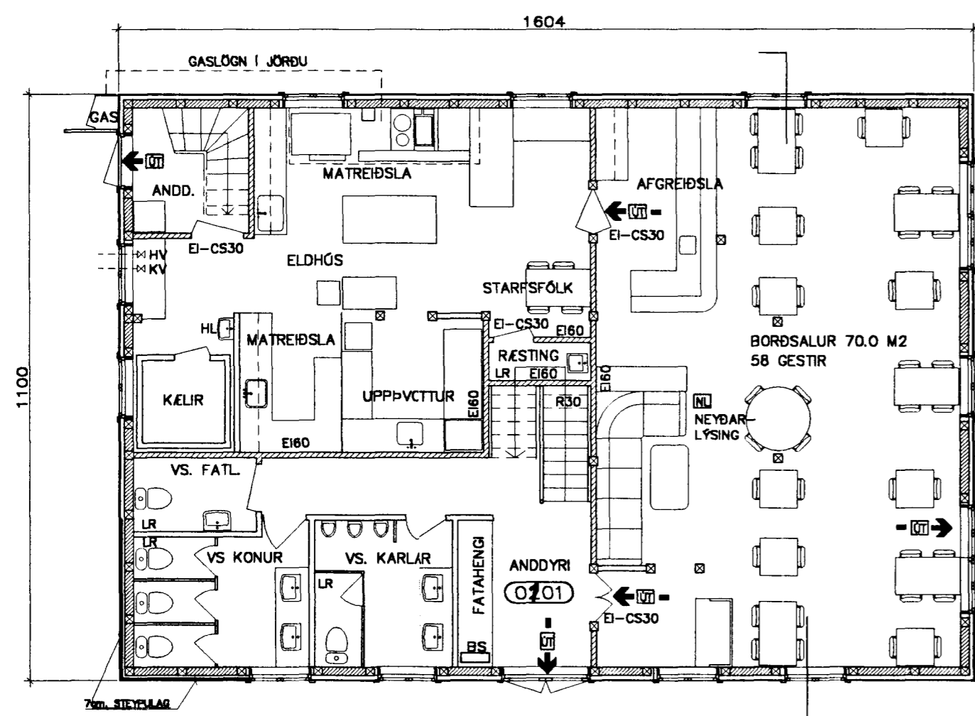
GRUNNMYND 1. HÆÐ
