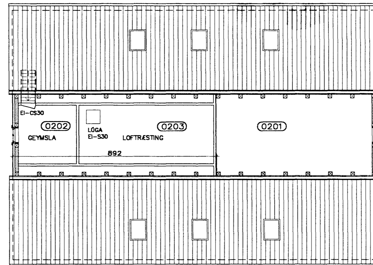
GRUNNMYND, RISHÆÐ
