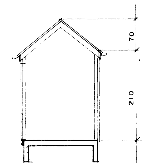
SKURÐUR 1:50
