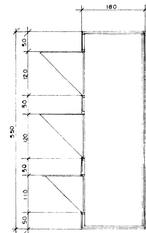
GRUNNMYND GEYMSLU 1:50
