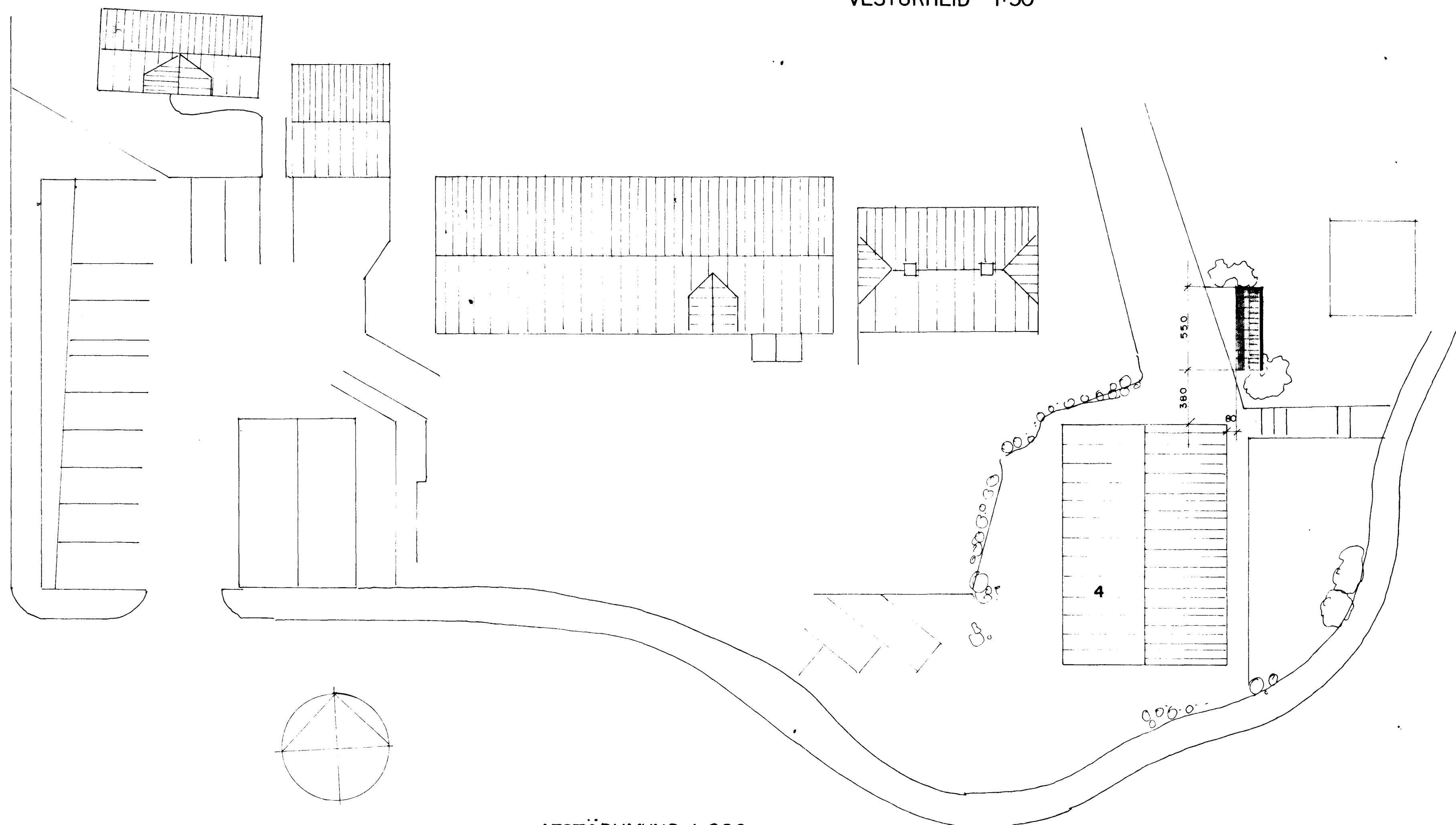
AFSTÖÐUMYND 1:200
