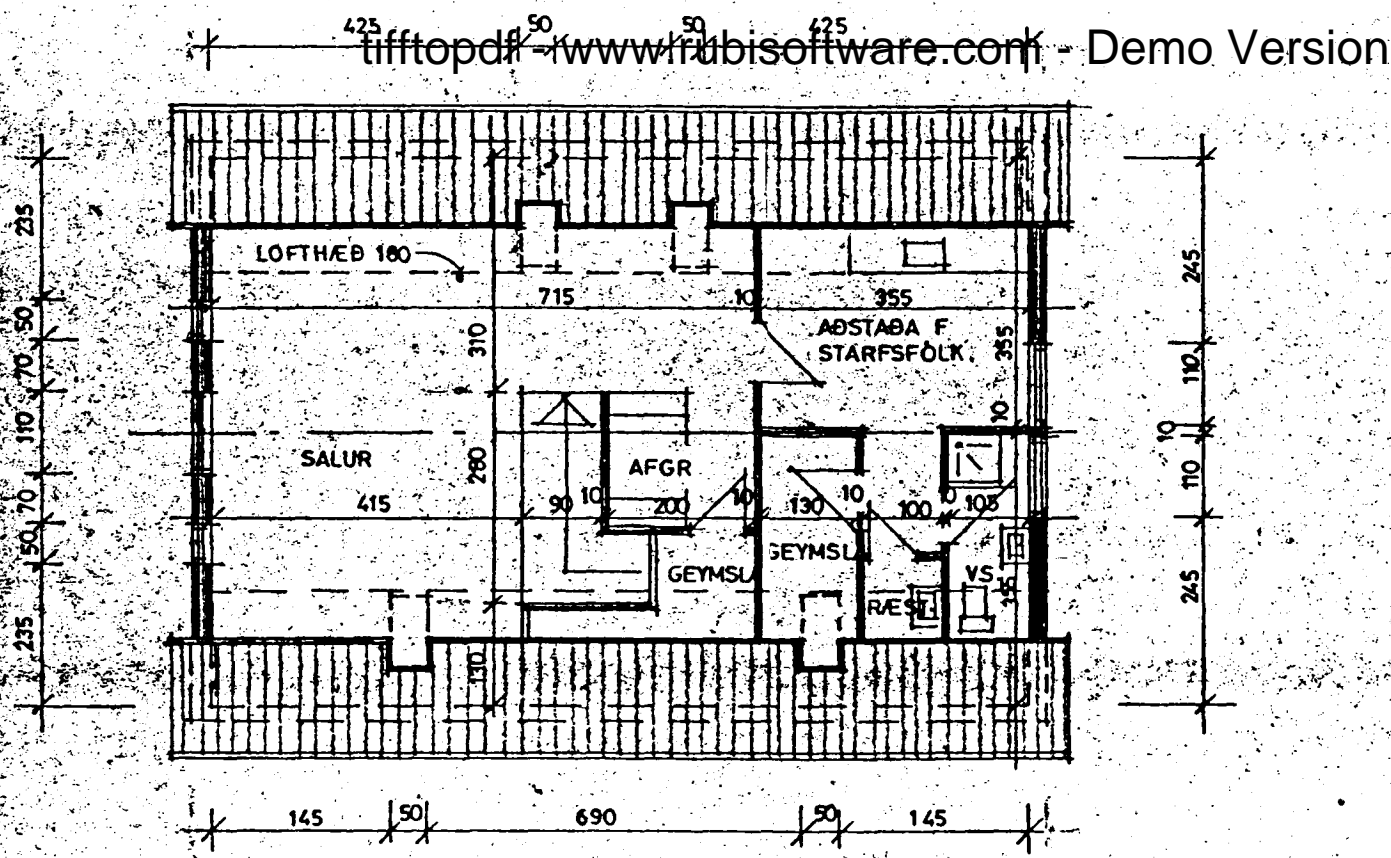
GRUNNMYND RISHÆÐAR 1:100
