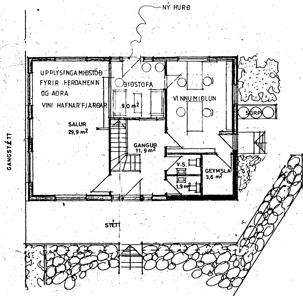
GRUNNMYND JARÐHÆÐAR 1:100
