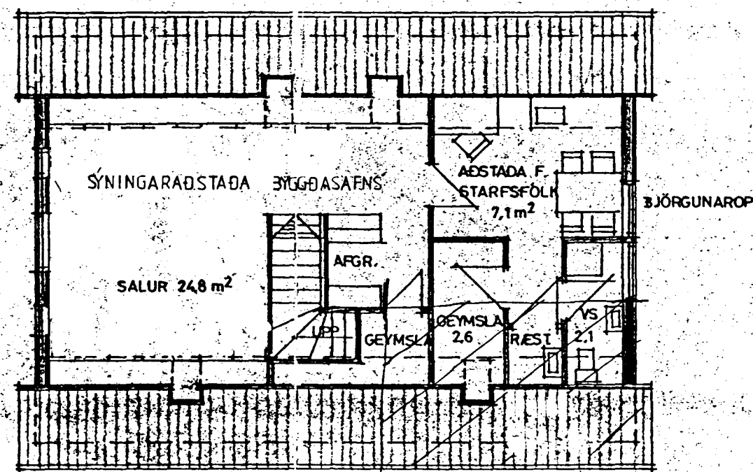
GRUNNMYND RISHÆÐAR 1:100
