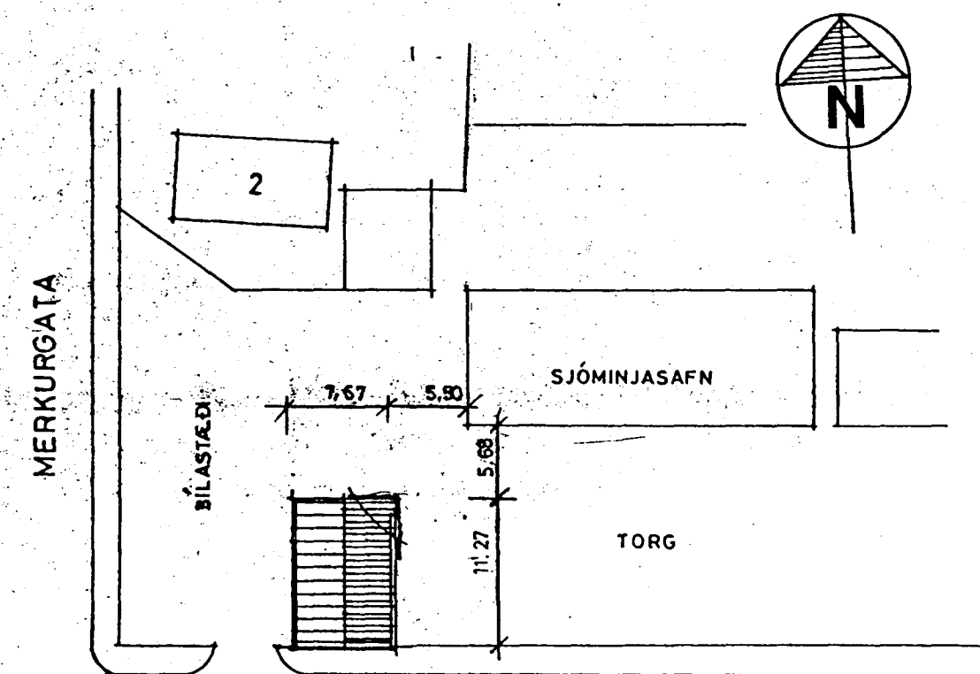
AFSTÖÐUMYND 1:500
