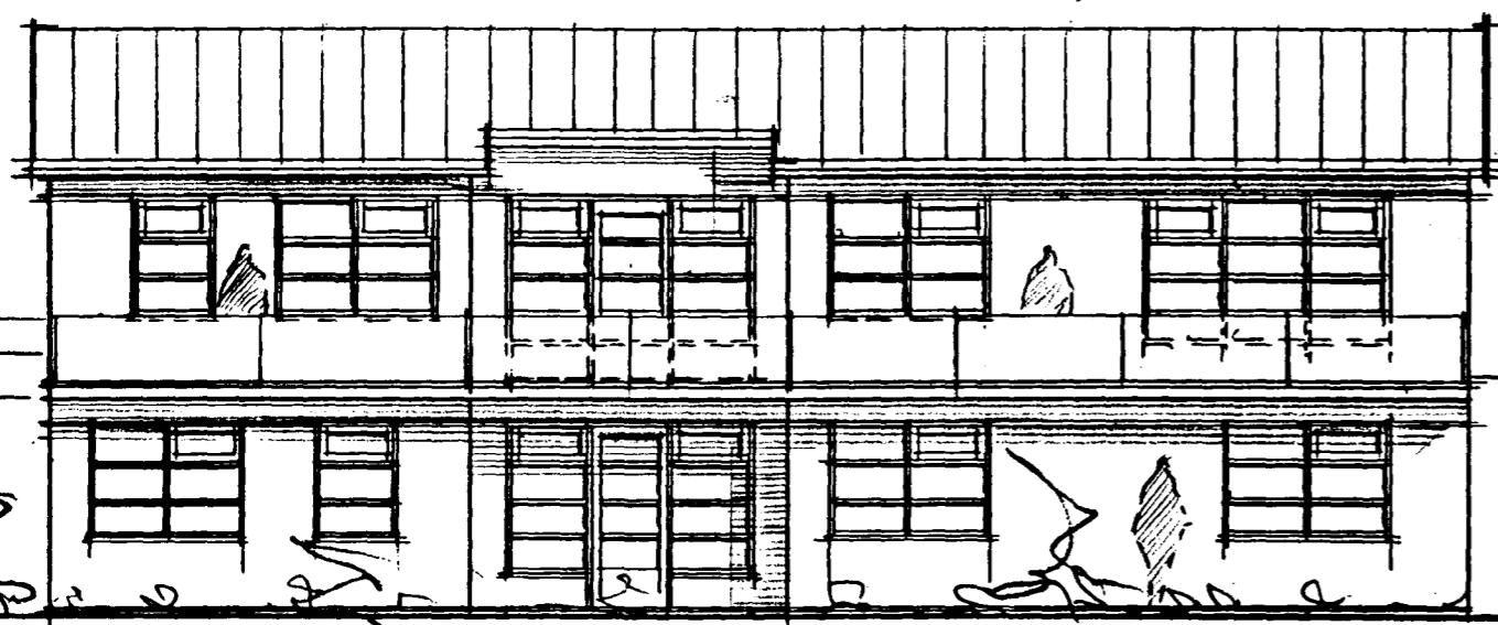
ÚTLIT SÚÐ-VESTUR M=1:100
