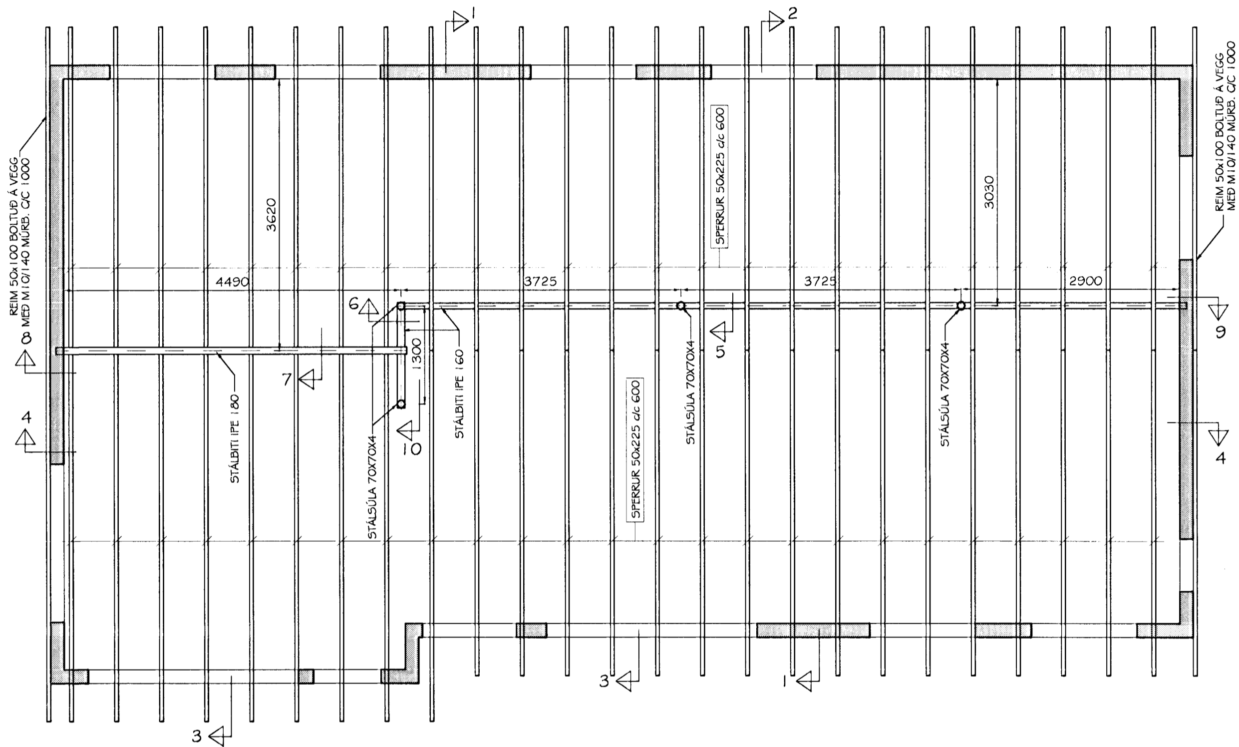
GRUNNMYND ÞAKVIÐA MKV. 1:50
