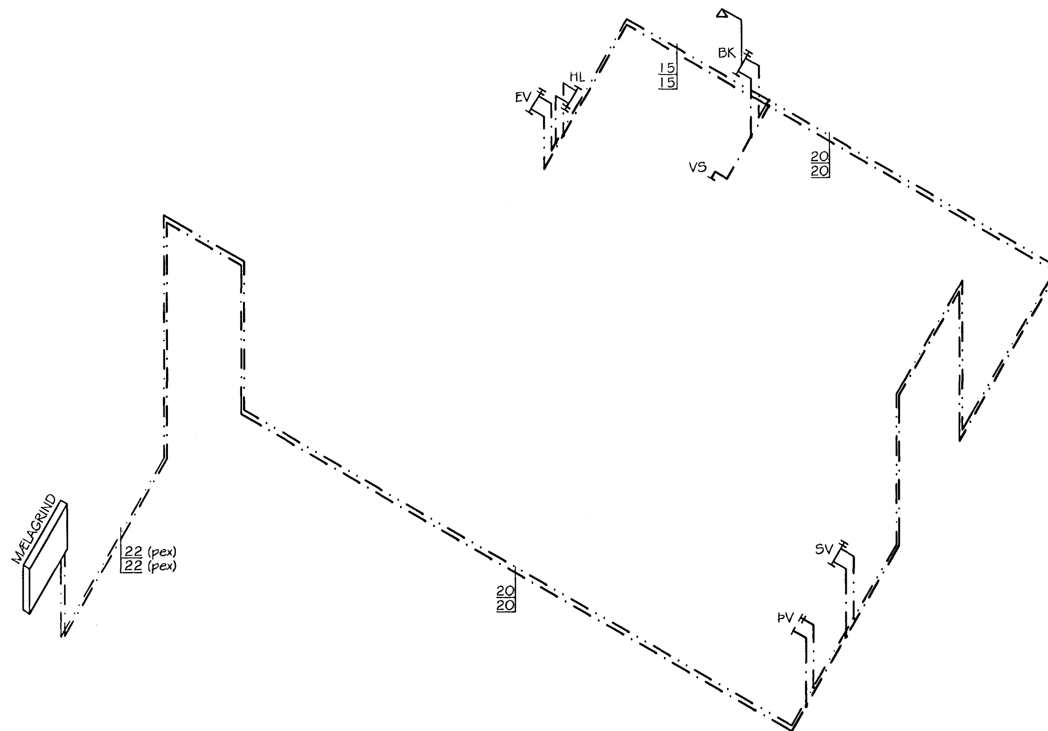
NEDRI HÆÐ RÚMMYND NEYSLUVATNSLAGNA MKV. 1:50
