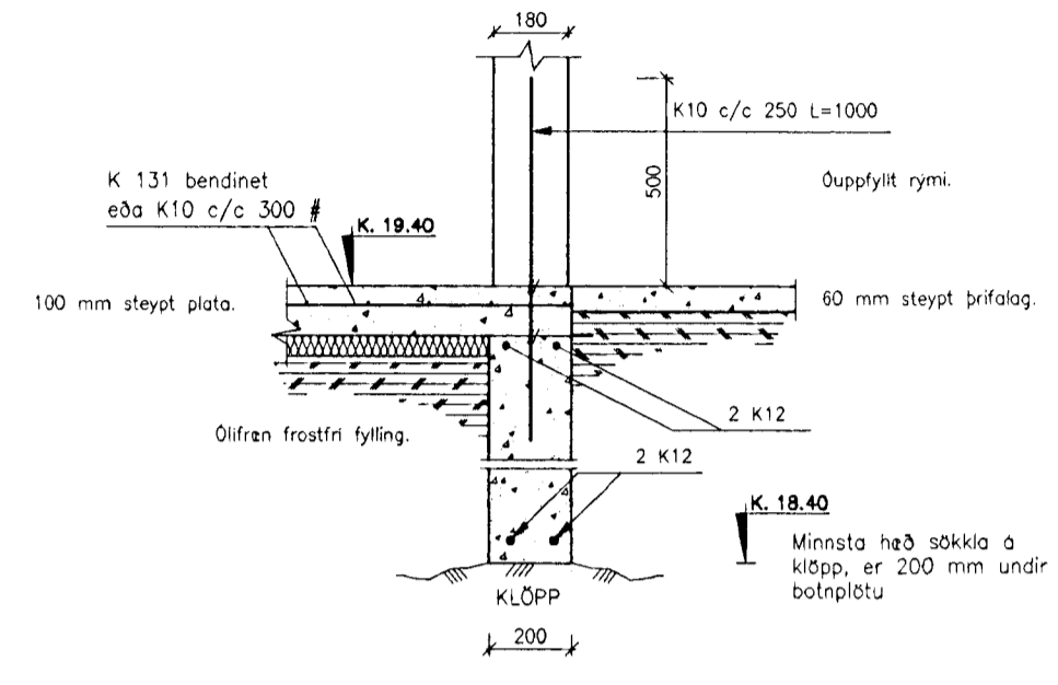
C Snið B 1 B 2 M. 1:20
