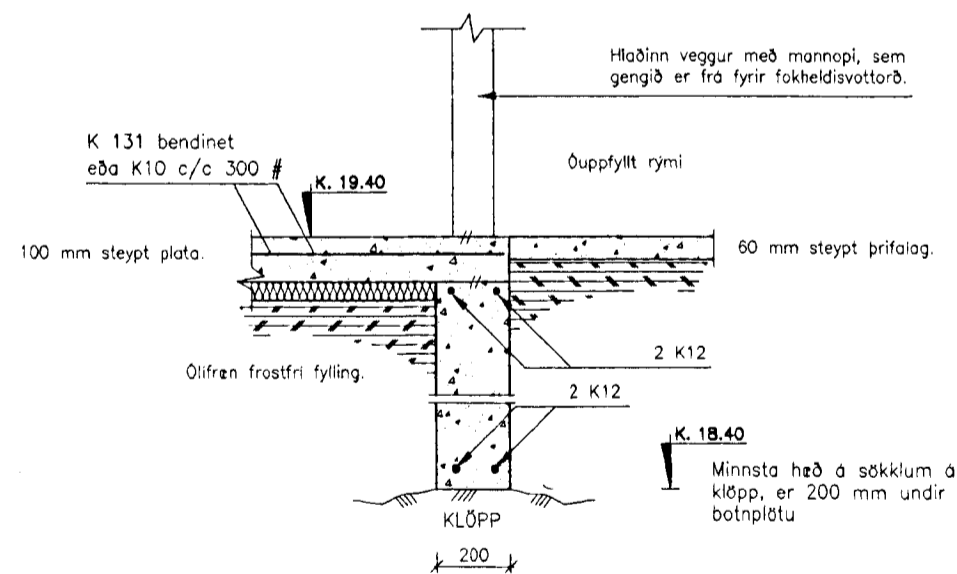
D Snið B 1 B 2 M. 1:20
