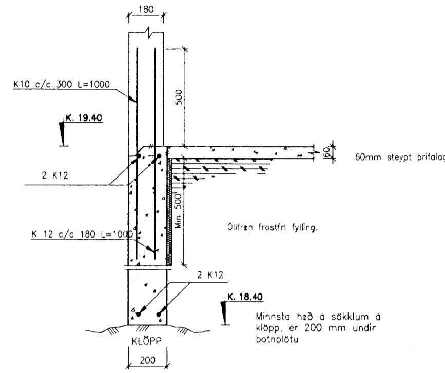
B Snið B 1 B 2 M. 1:20
