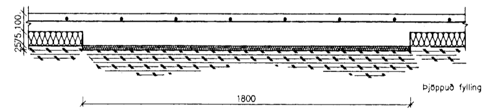
E Snið B 1 B 2 M. 1:20
