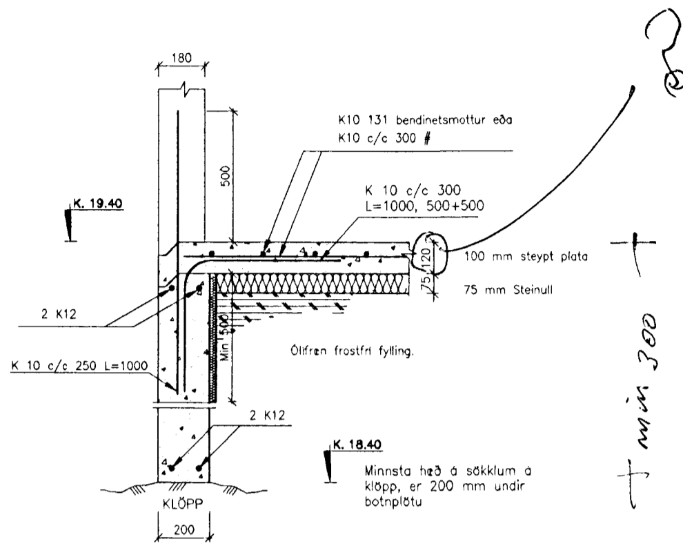
A Snið B 1 B 2 M. 1:20
