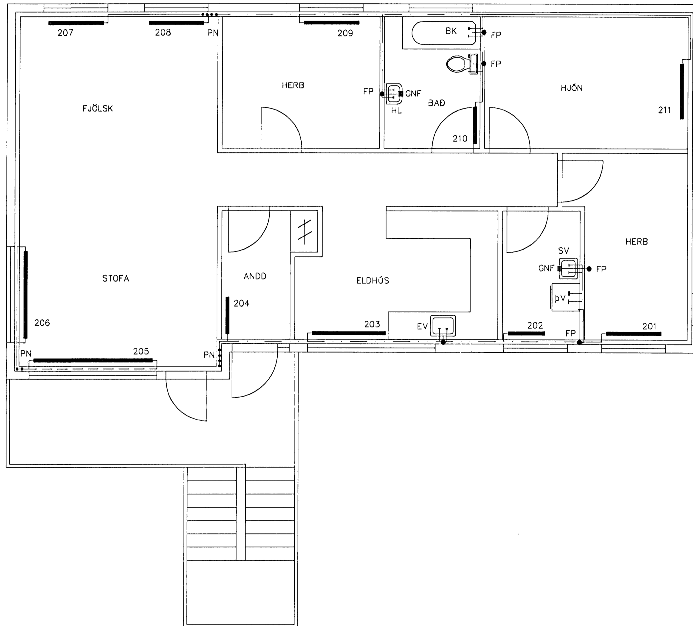
GRUNNMYND 2 HÆÐAR 1:50
