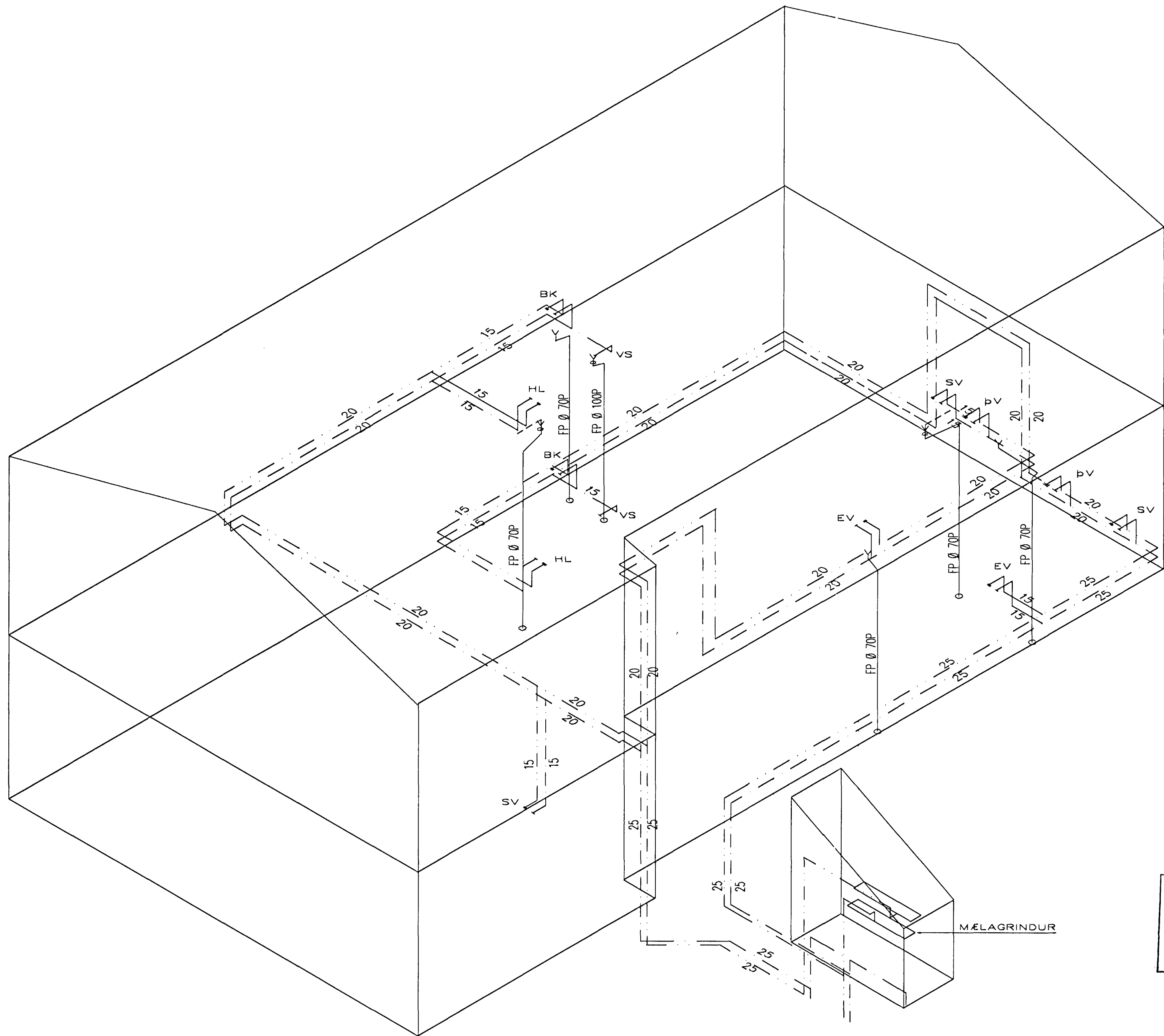
RÚMMYND VATNS OG FRÁRENNSLISLAGNA 1:50
