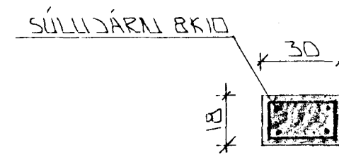
SÚLA S3 • 1:20
