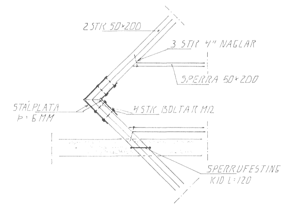
DEILI 4.1:20
