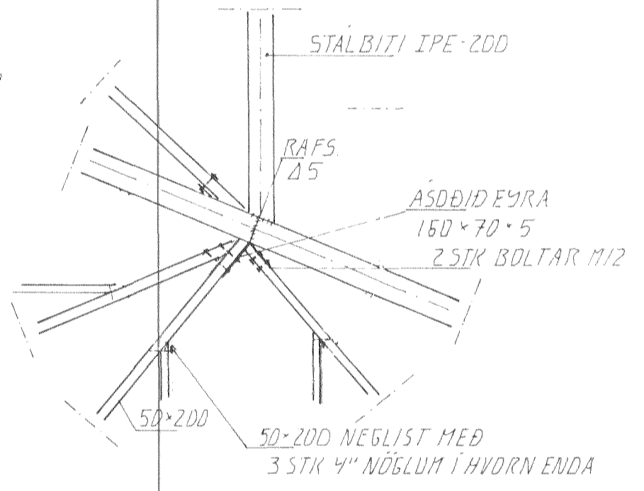
DEILI 3.1:20
