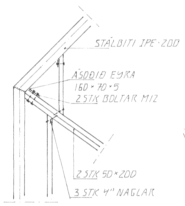
DEILI 2.1:20
