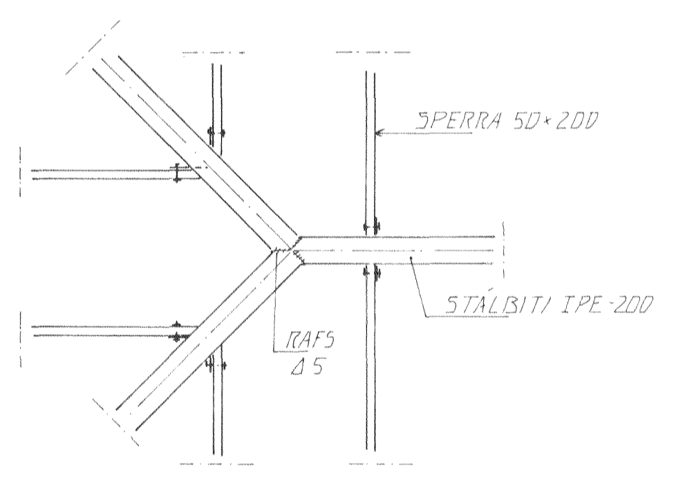
DEILI 1.1:20
