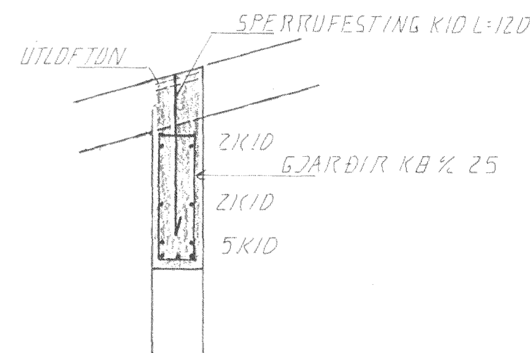
SNIÐ 4. 1:20
