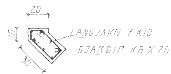
SÚLA 1. 1:20
