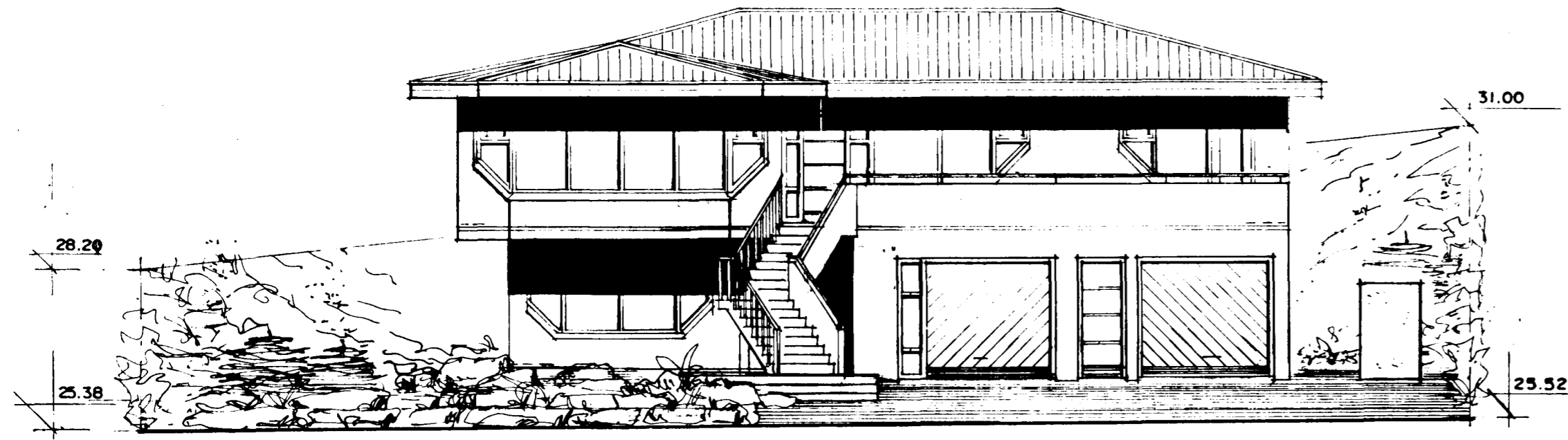
SUÐVESTUR MKV. 1:100
