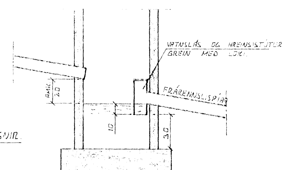
VATNSLÁS OG HREINISSTÖTUR BREIN MED LÖGI FRÁRENNISPIPA BRUNNUR ÞEIR DREYPTU OG REGNURTU FRÁRENNISPIPA SIGAL VERR AMK 150 CM. FRÁ ÞEIRISKRI DREYVEGS
