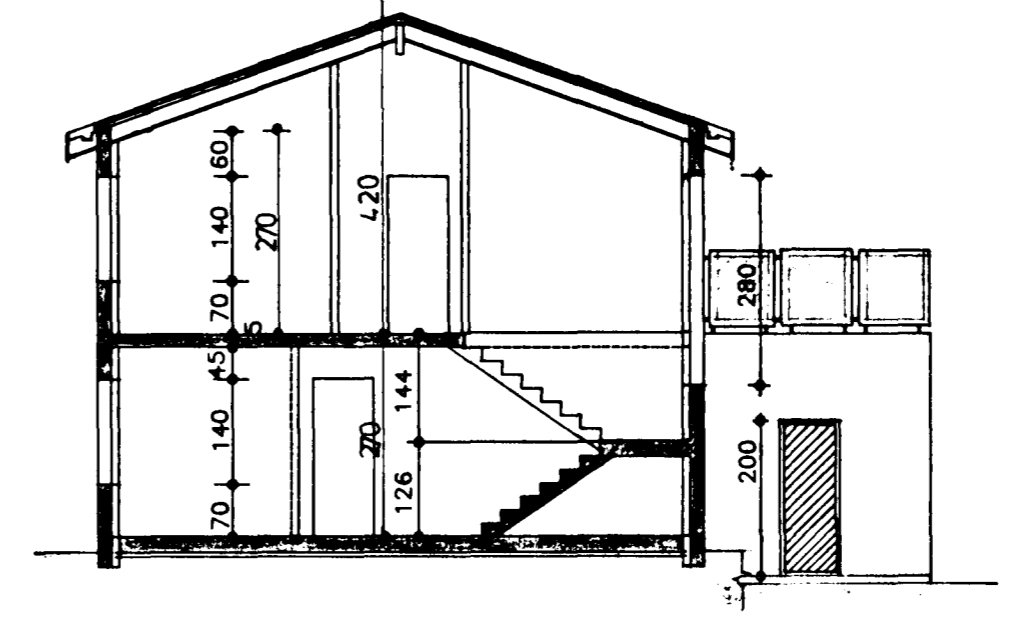
SNID A-A
