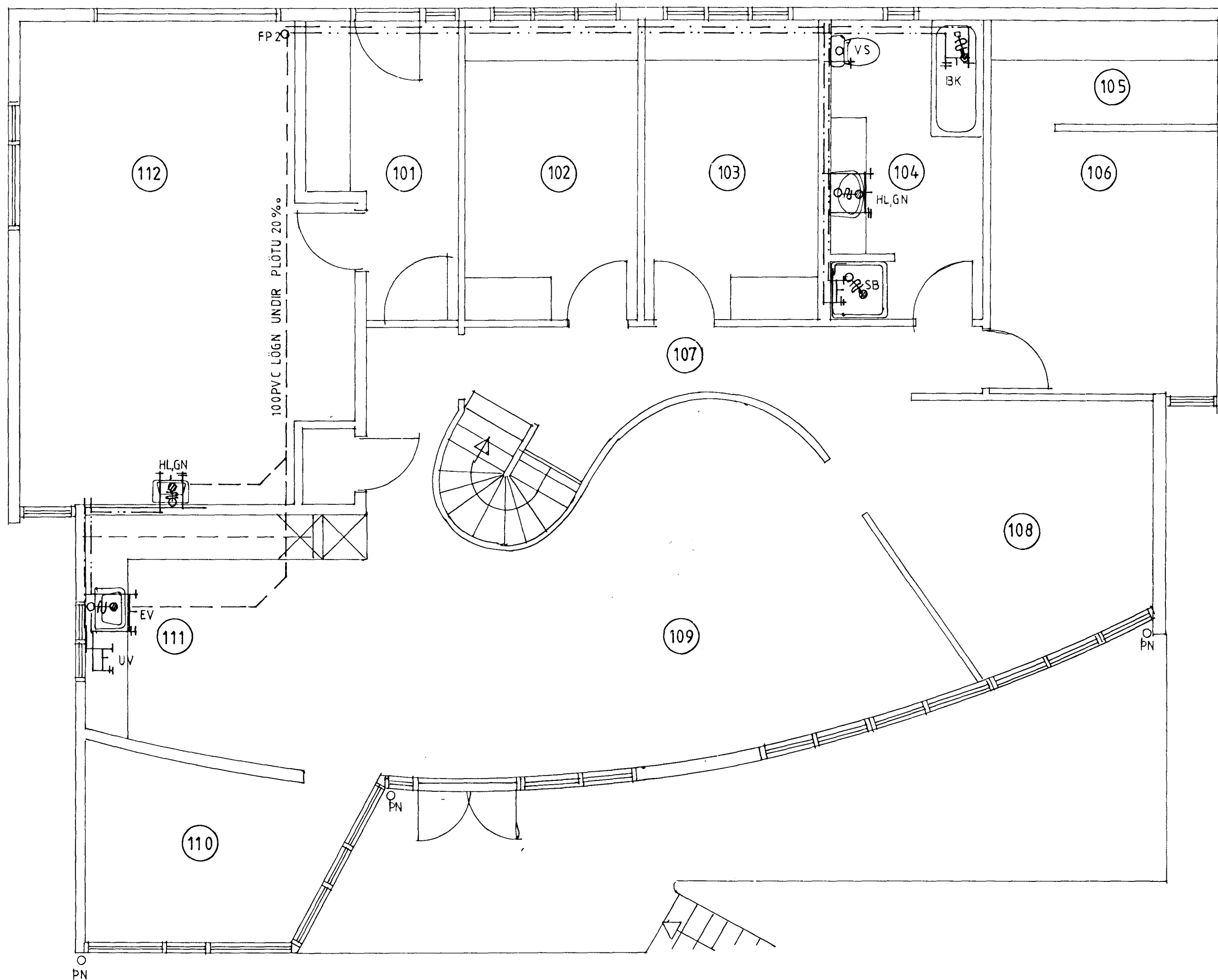
GRUNNMYND EFRI HÆÐAR 1:50
