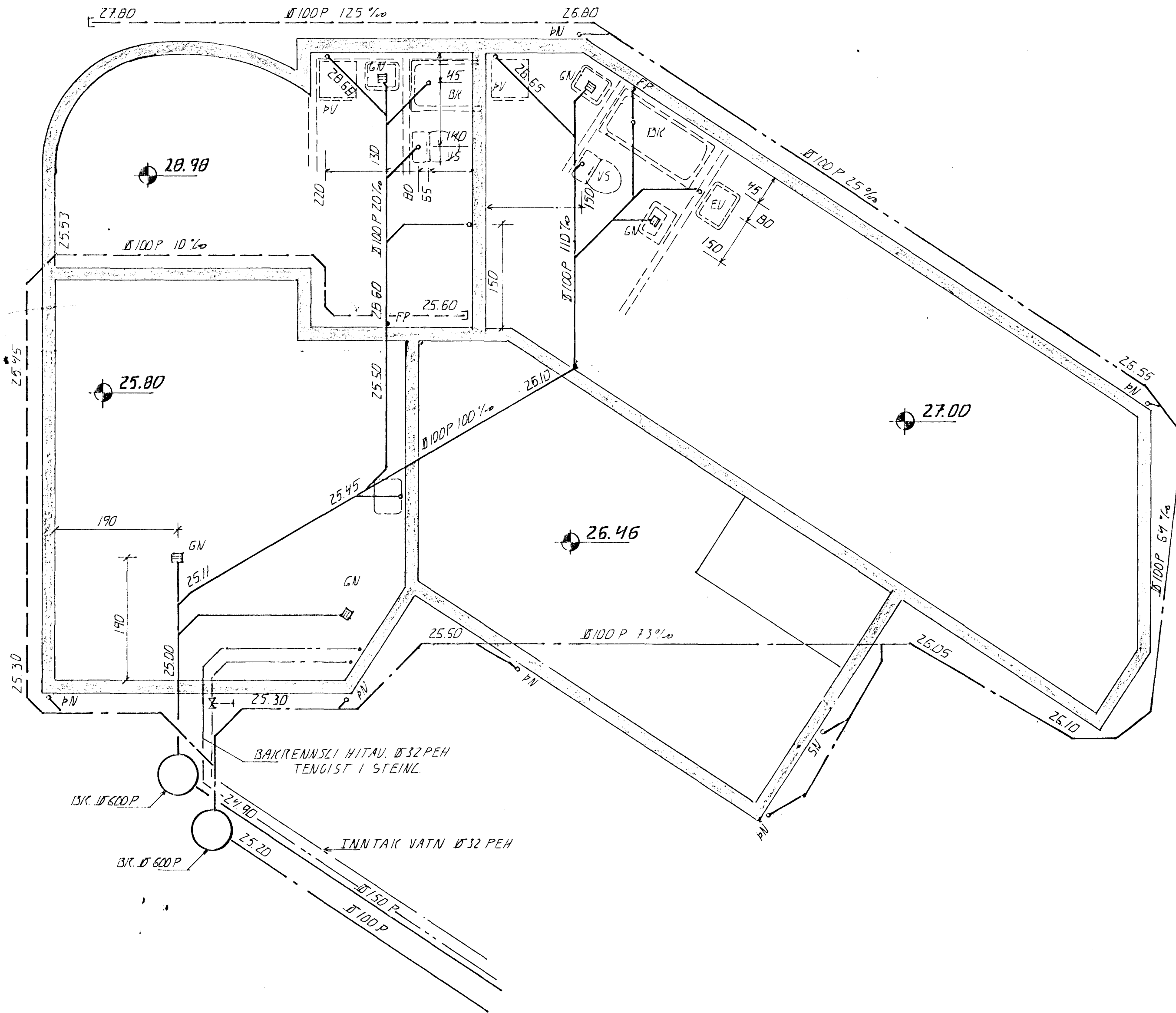
GRUNNMÝND, 1:50
