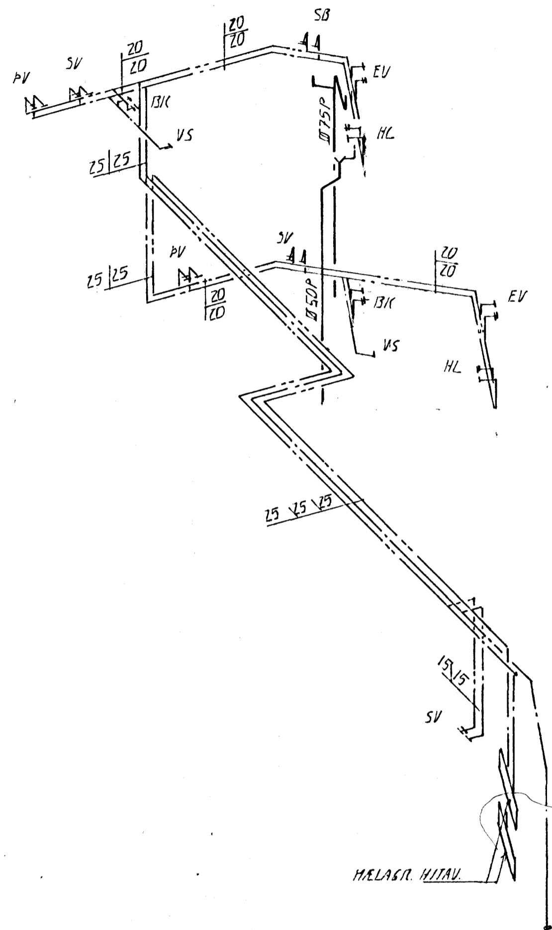
VATNS- OG FRÁRENNSLISLAGNIR. 1:50
