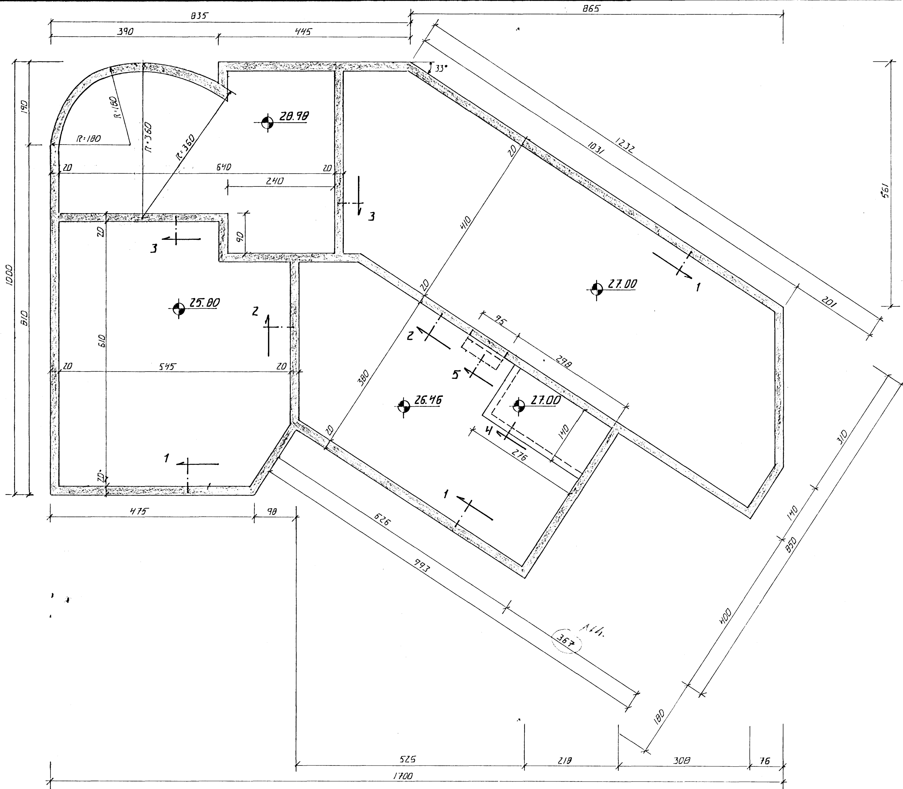
GRUNNMÖND . 1:50
