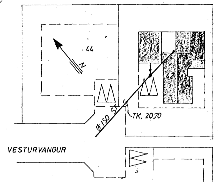
AFSTAÐA 1:500
