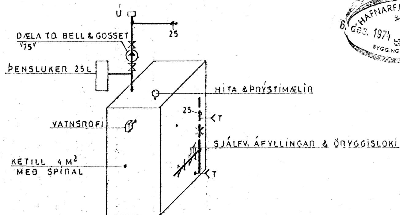
TENGIMYND VIÐ KÉTIL
