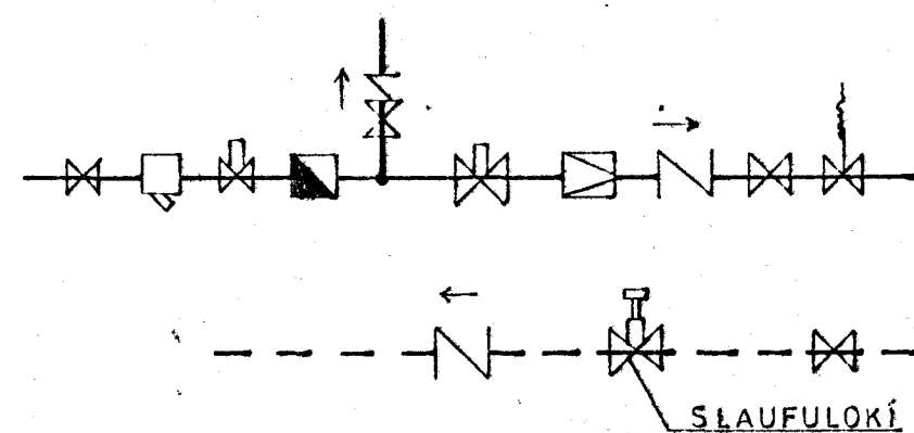
TENGIMYND VIÐ MÆLAGRIND
