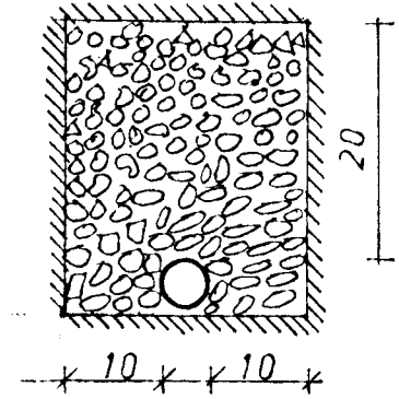
JARÐVATNSLÖGN ÞVERSNÍÐ 1:10
