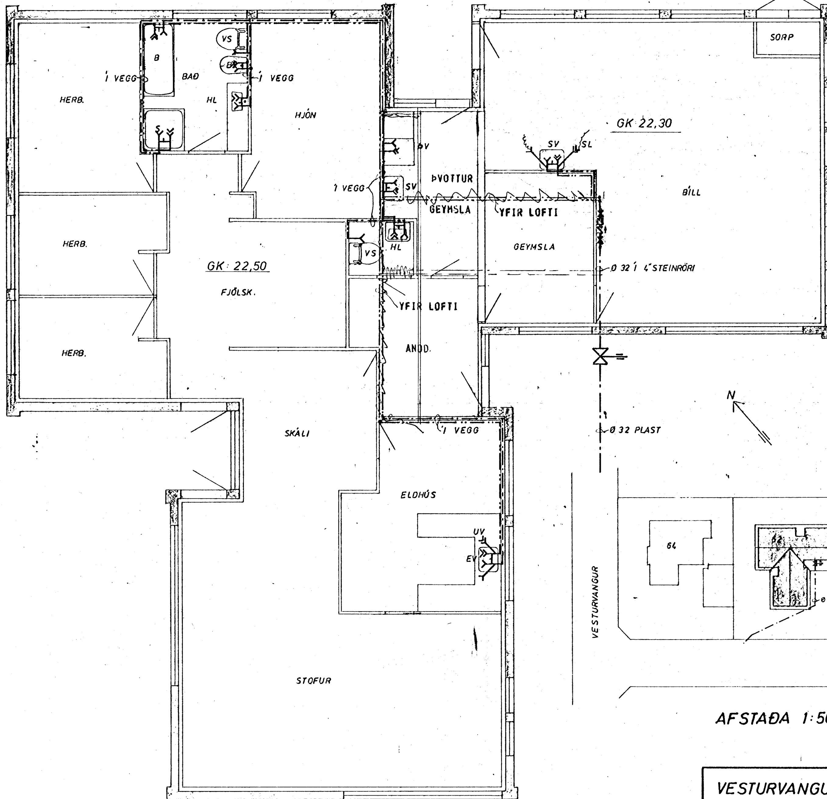
GRUNNMYND 1:50
