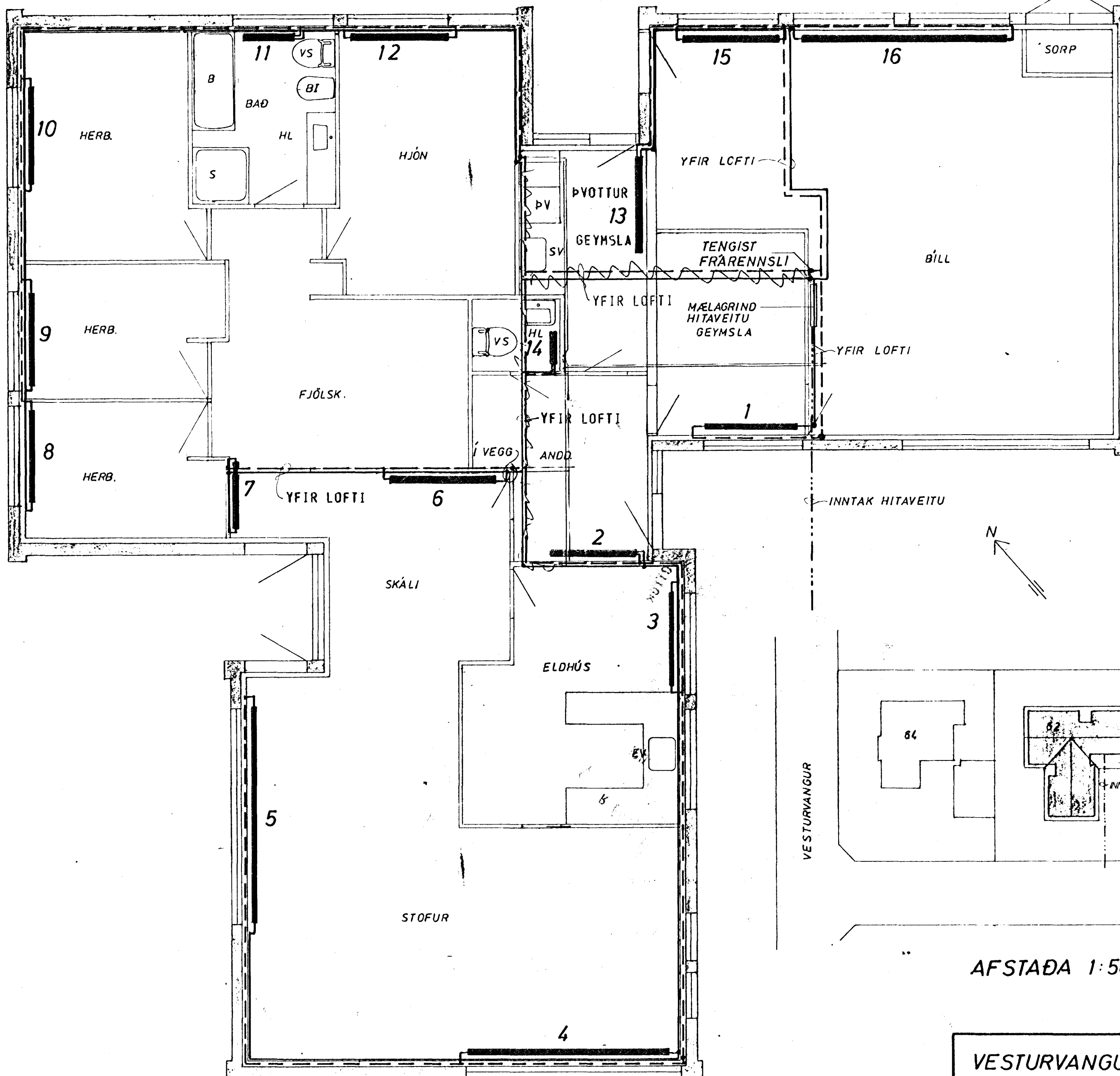
GRUNNMYND 1:50
