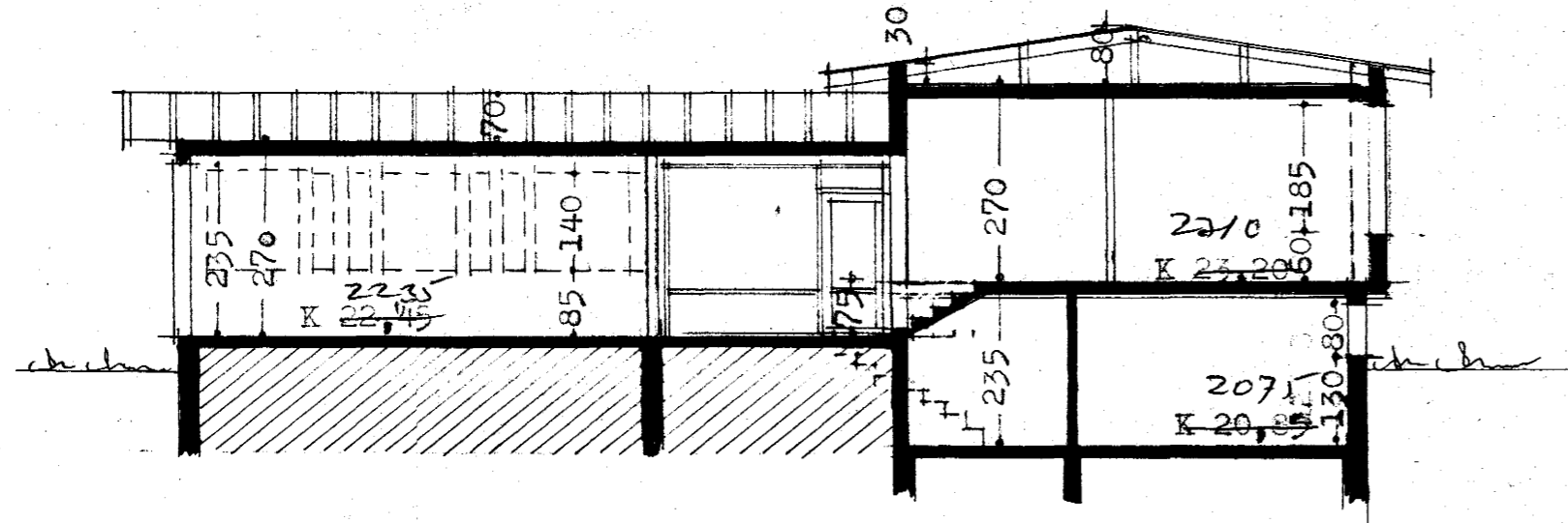
skurður A - A
