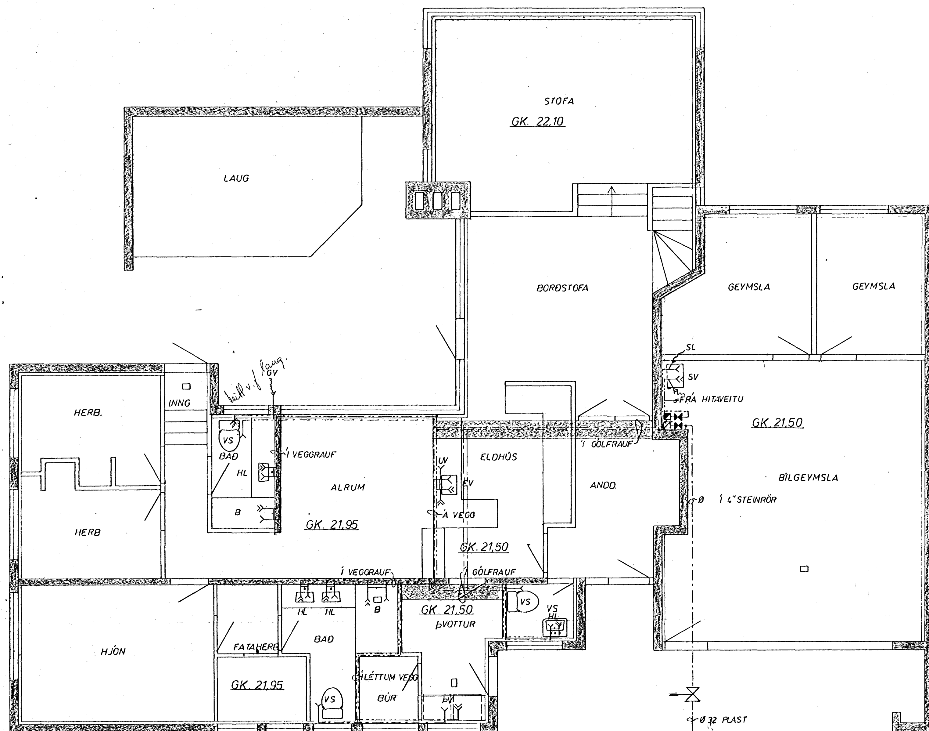
GRUNNMYND 1:50
