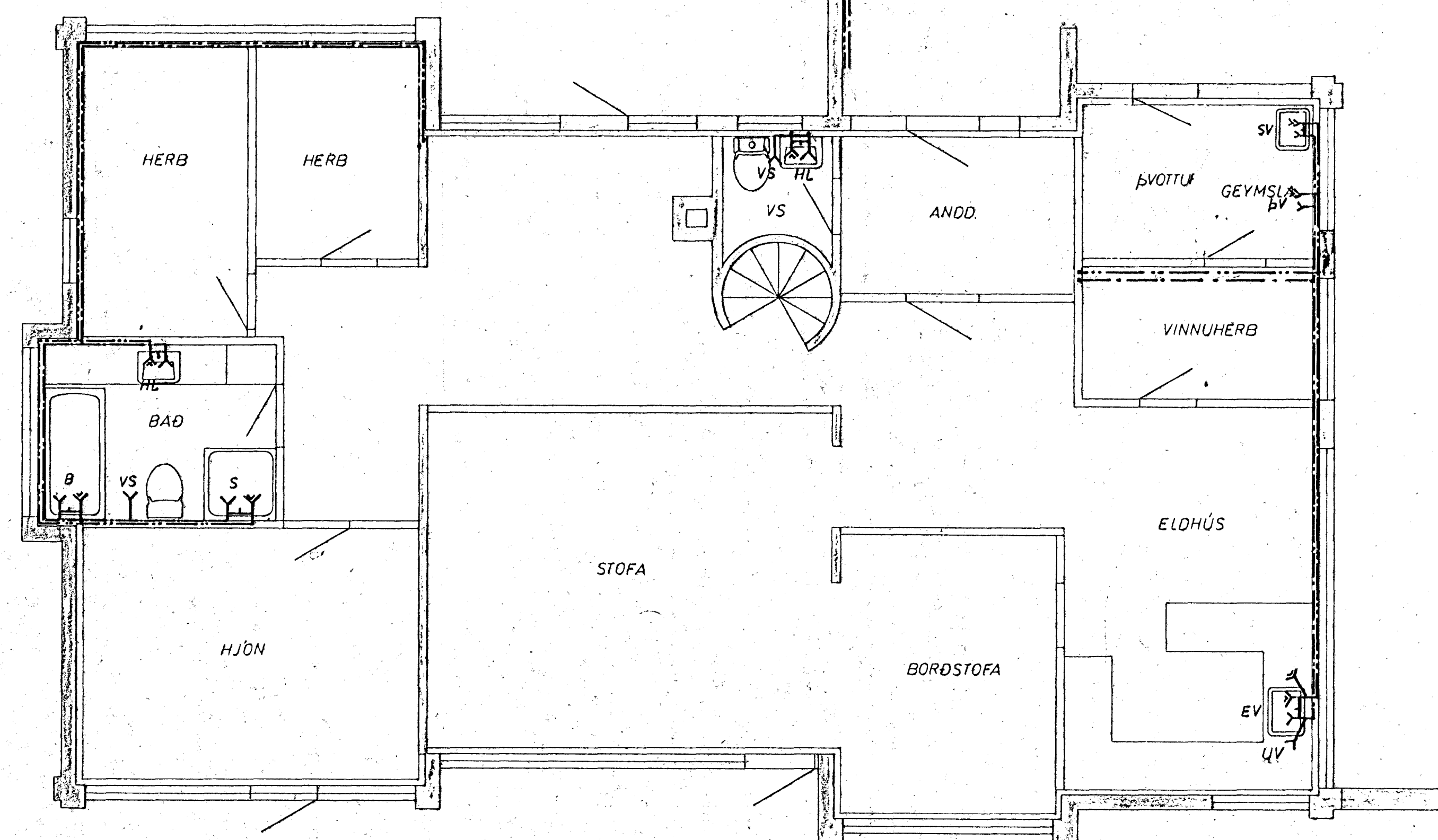
GRUNNMYND 1:50
