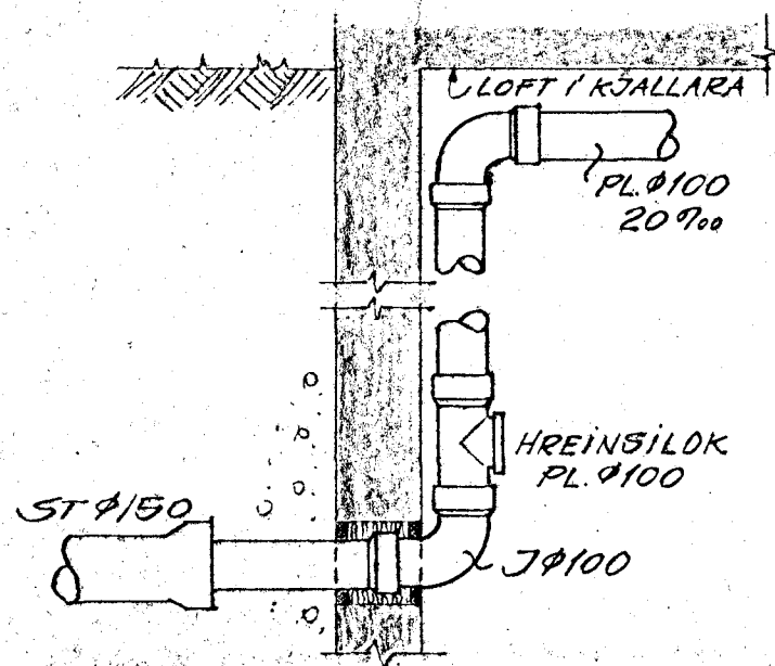
SNÍÐ A-A. 1:20
