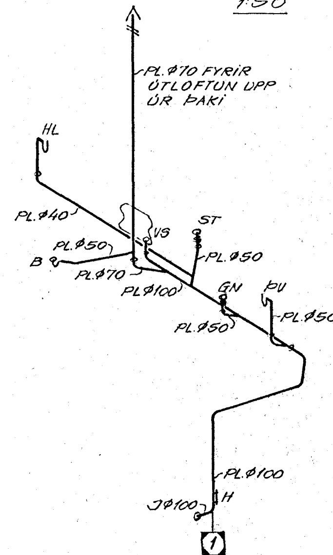
RÚMMYND AF STOFNI 1:50
