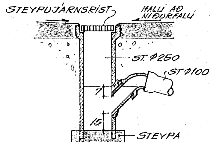
GN. Í BÍLSKÚR. 1:20
