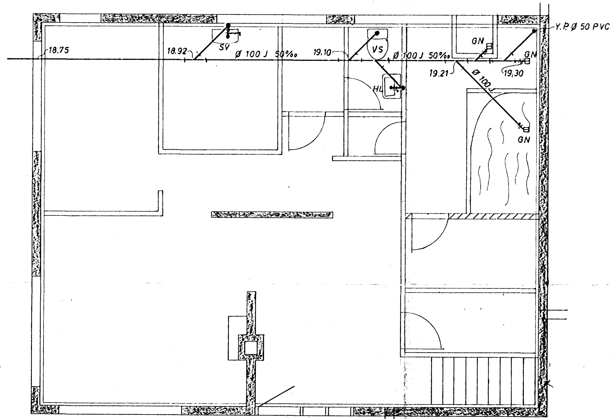
GRUNNMYND KJALLARA 1:50
