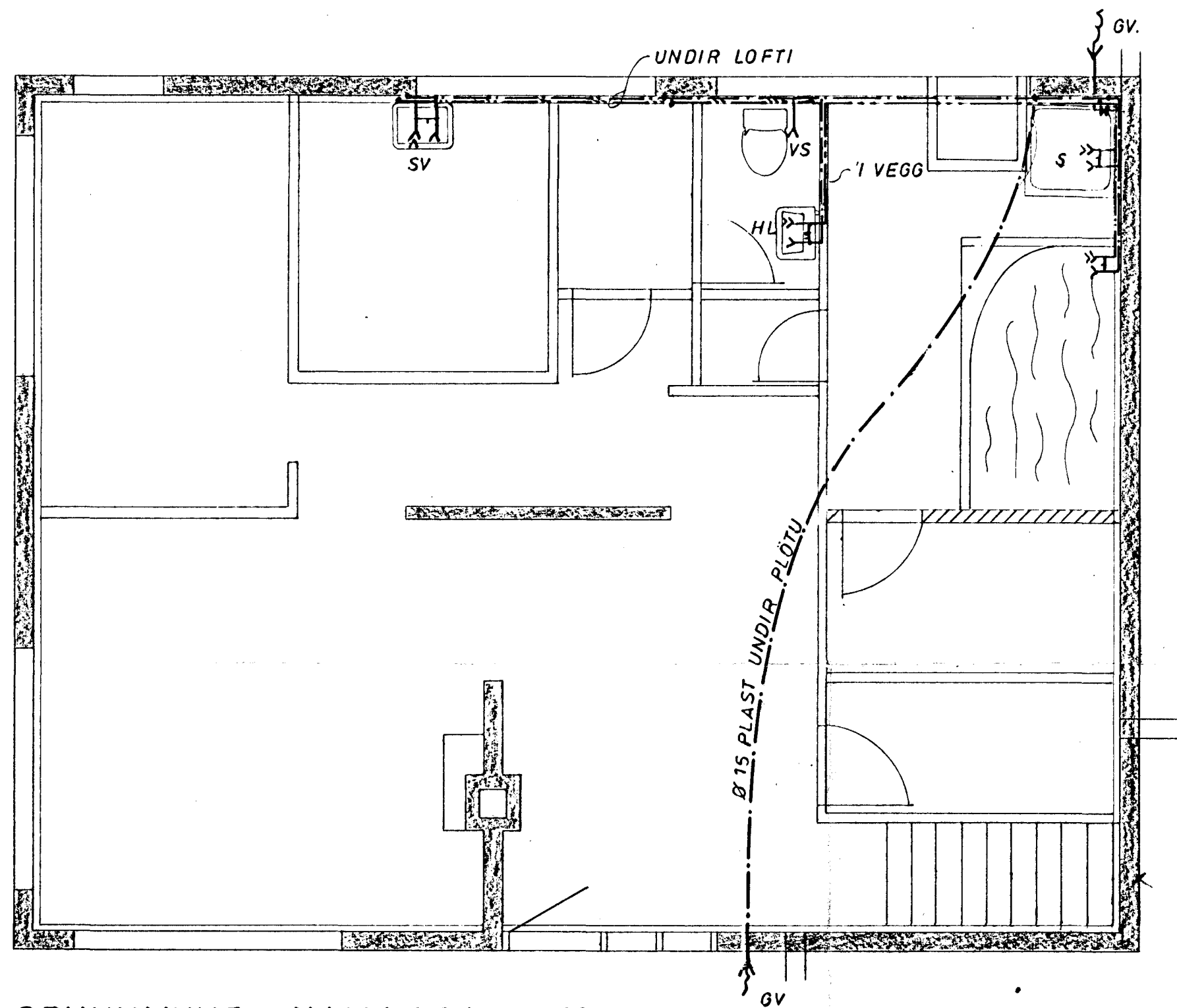
GRUNNMYND KJALLARA 1:50
