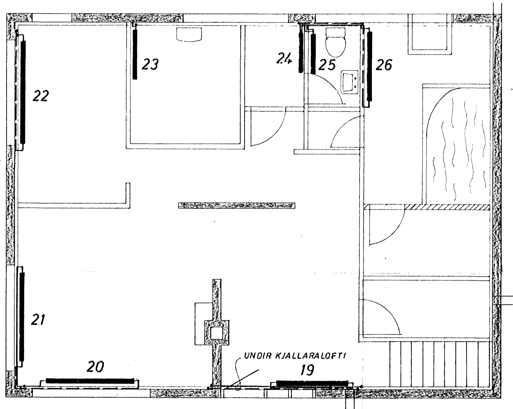
GRUNNMYND KJALLARA 1:50
