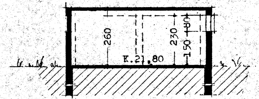
Skurður B-B
