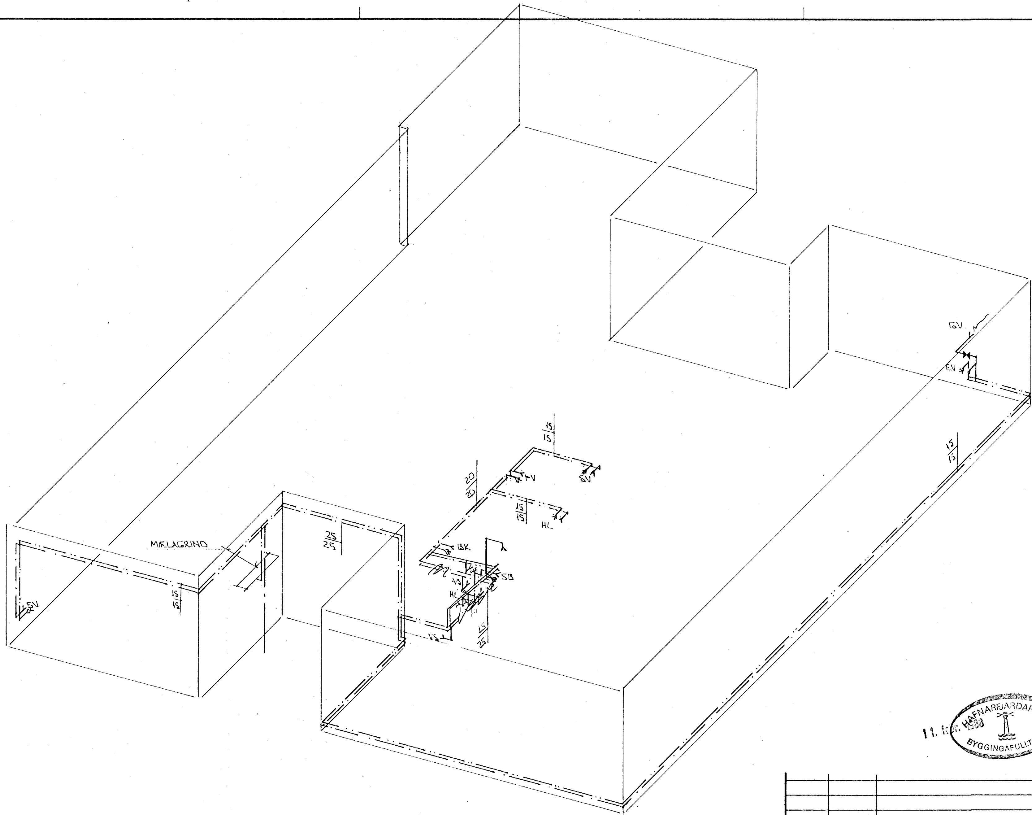
RÚMMYND VATNSLAGNA 1:50
