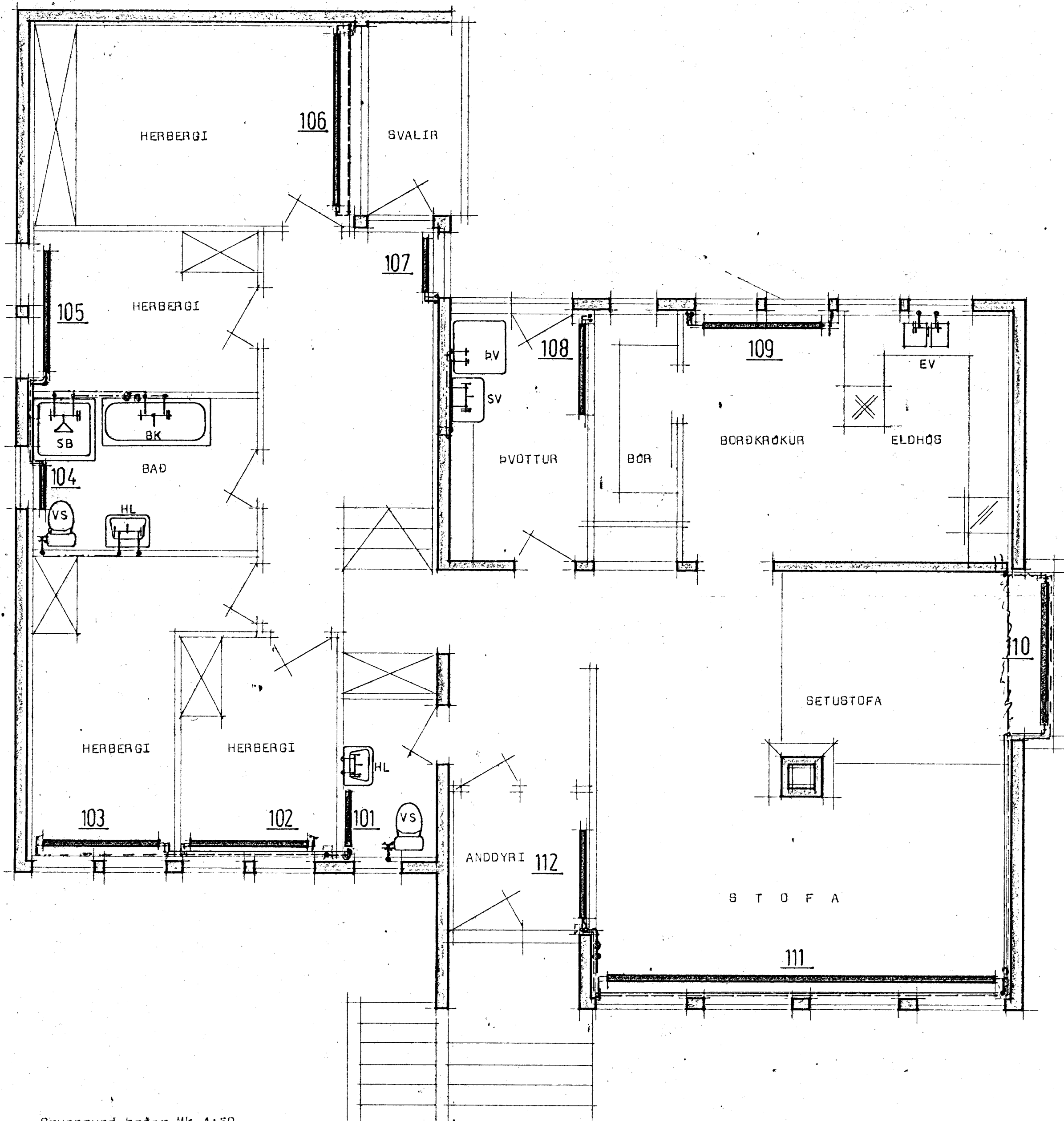
Grunnmynd hæðar MK 1:50
