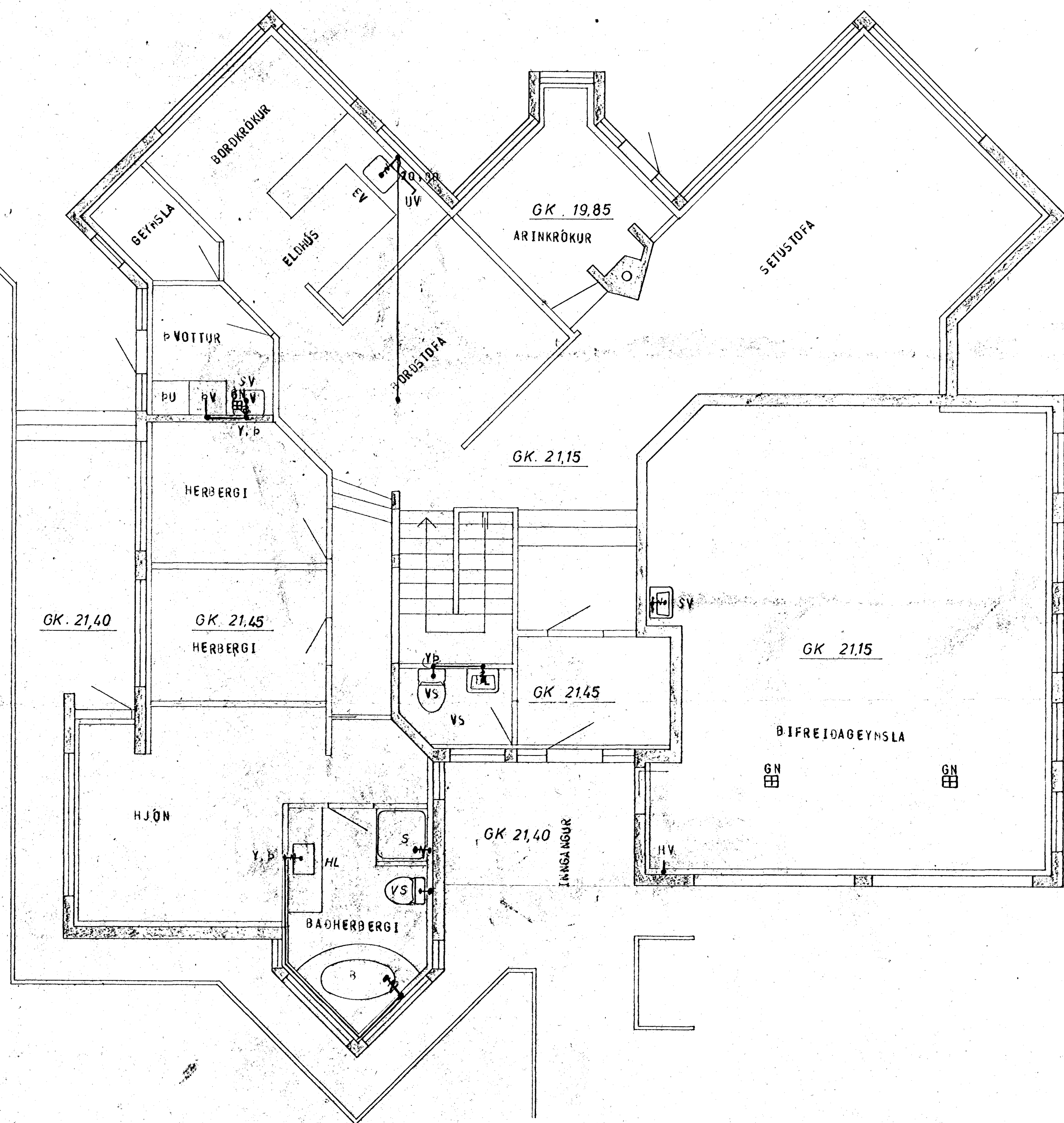
GRUNNMYND HÆÐAR 1:50
