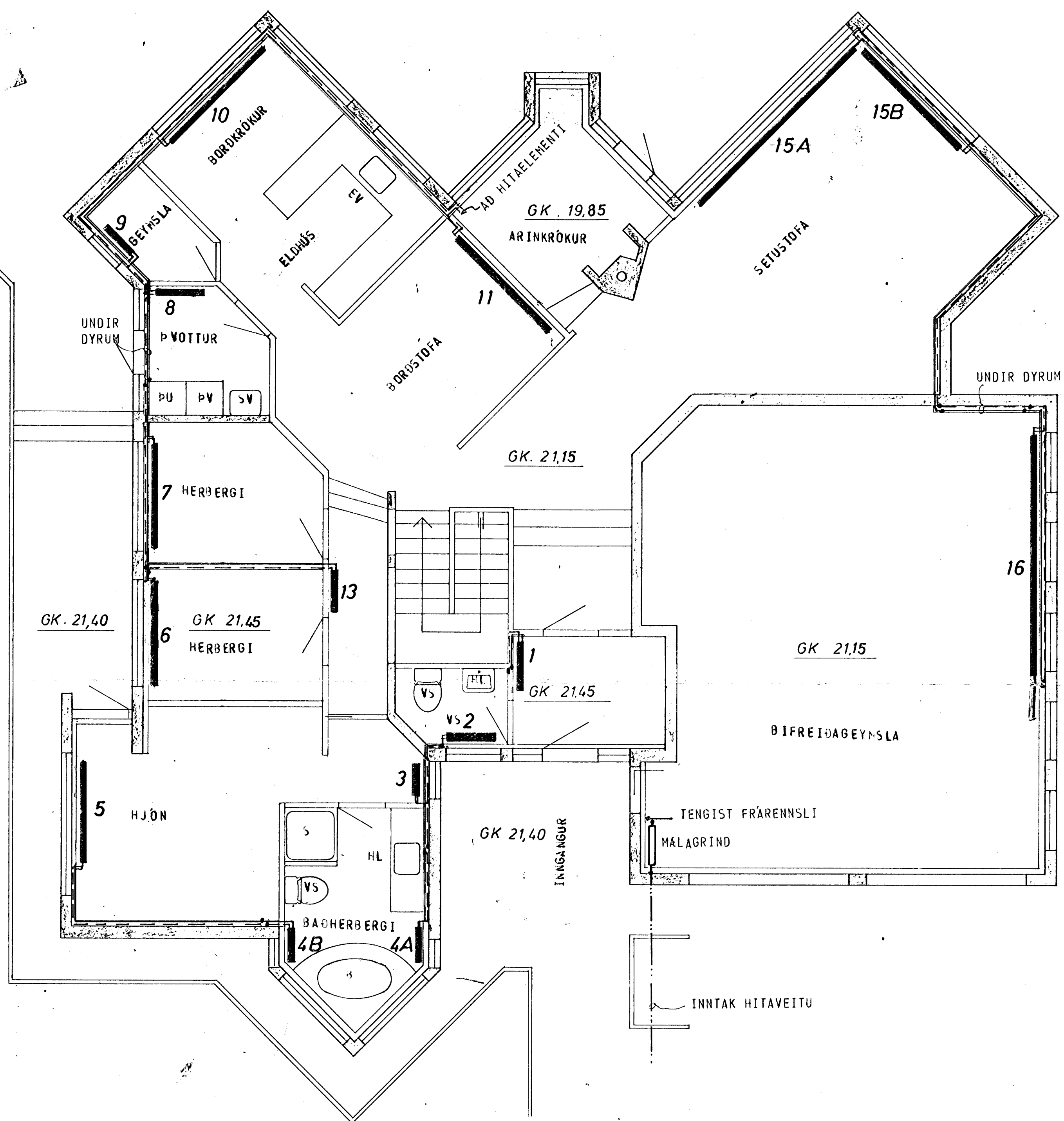
GRUNNMYND HÆÐAR 1:50
