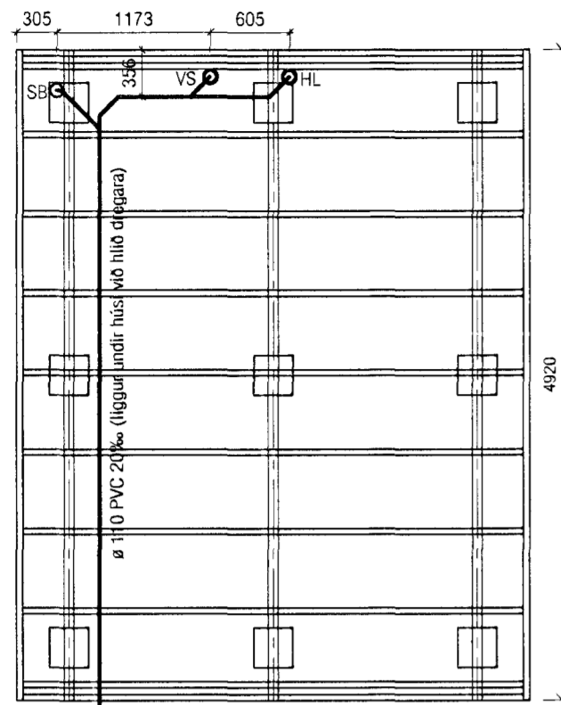
Grunnmynd, húsagerð A. 1:50
