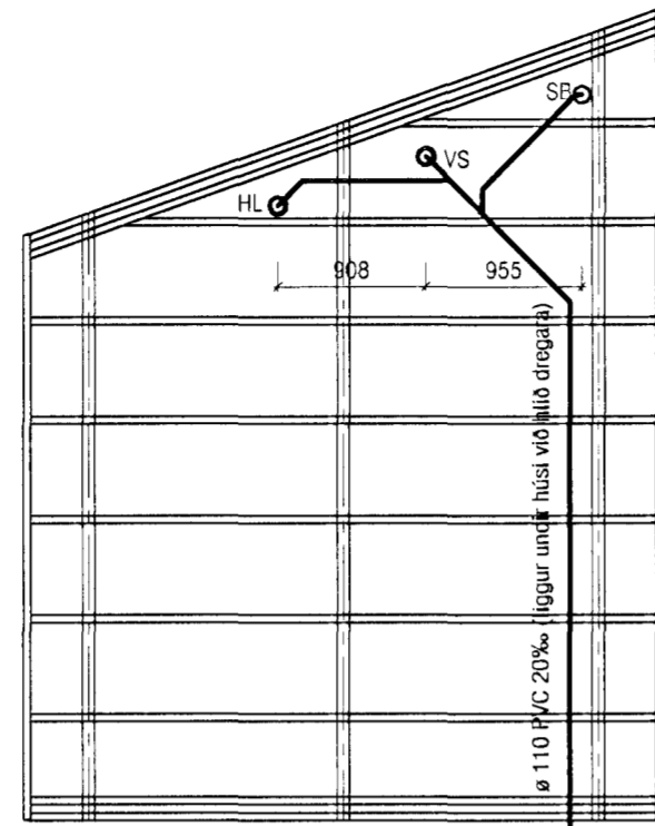
Grunnmynd, húsagerð B. 1:50
