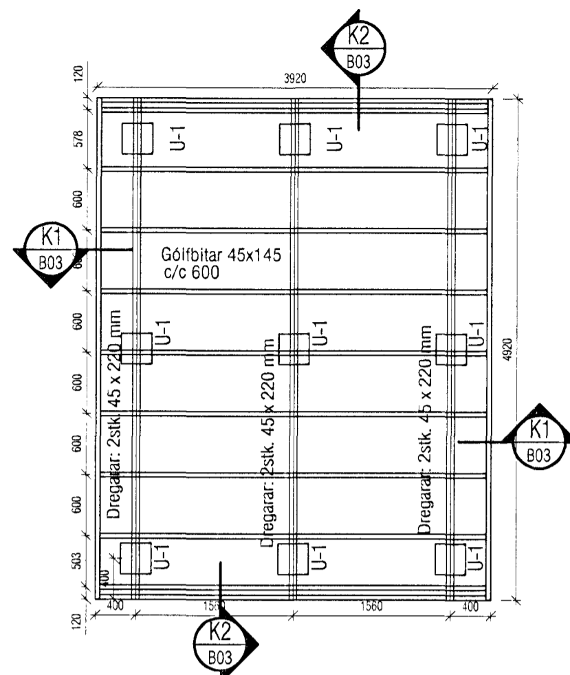
Gólfbitar, grunnmynd 1:50
