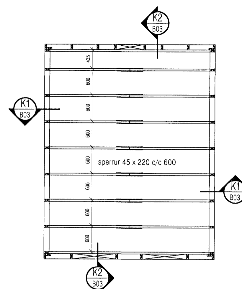
Þakvirki, grunnmynd 1:50
