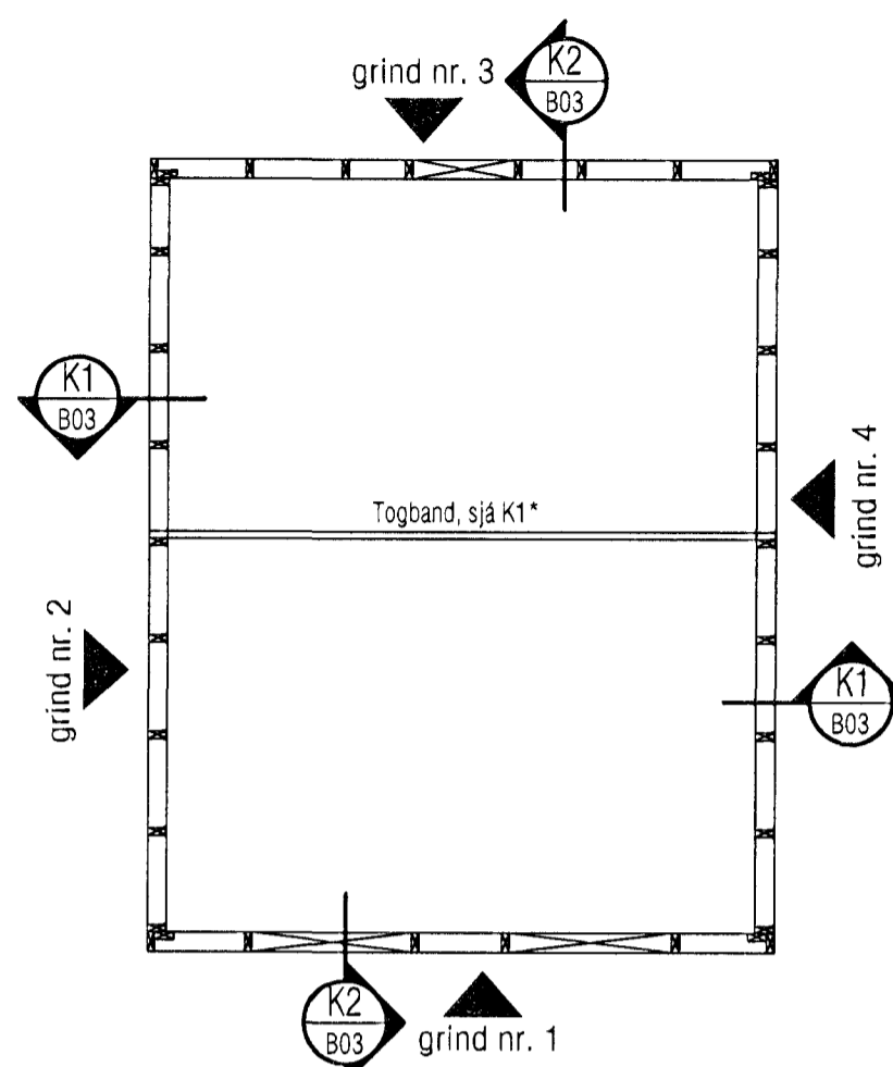
Veggjagrindur, grunnmynd 1:50
