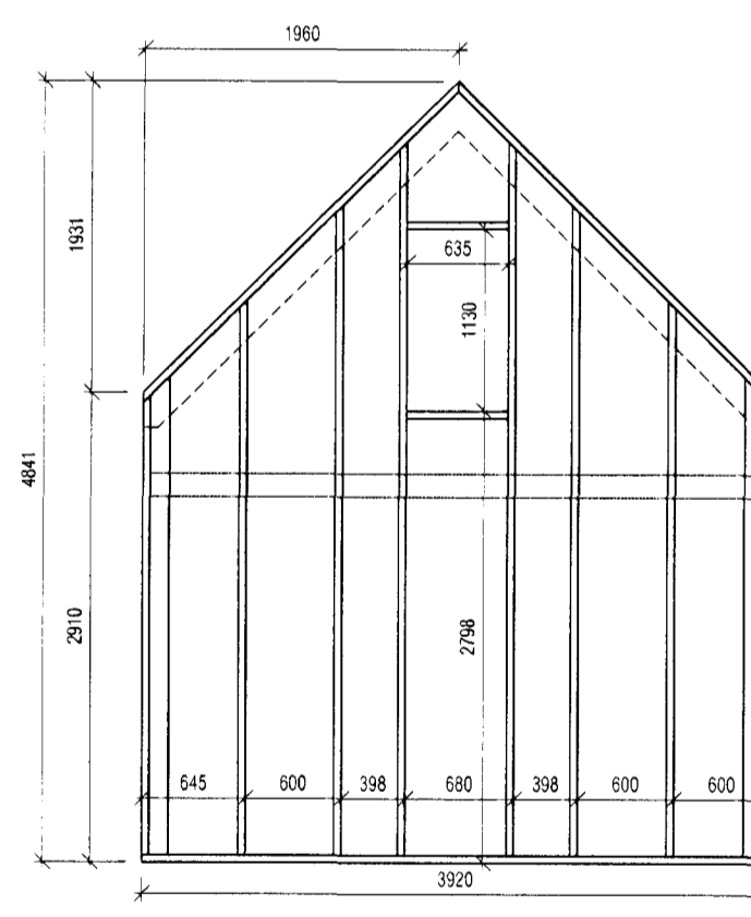
grind nr. 3
