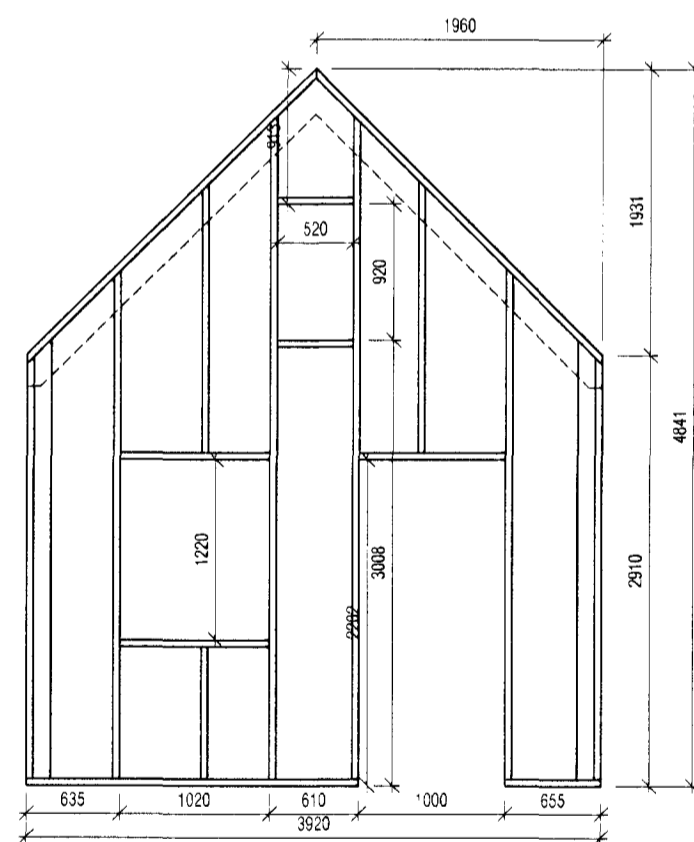
grind nr. 1
